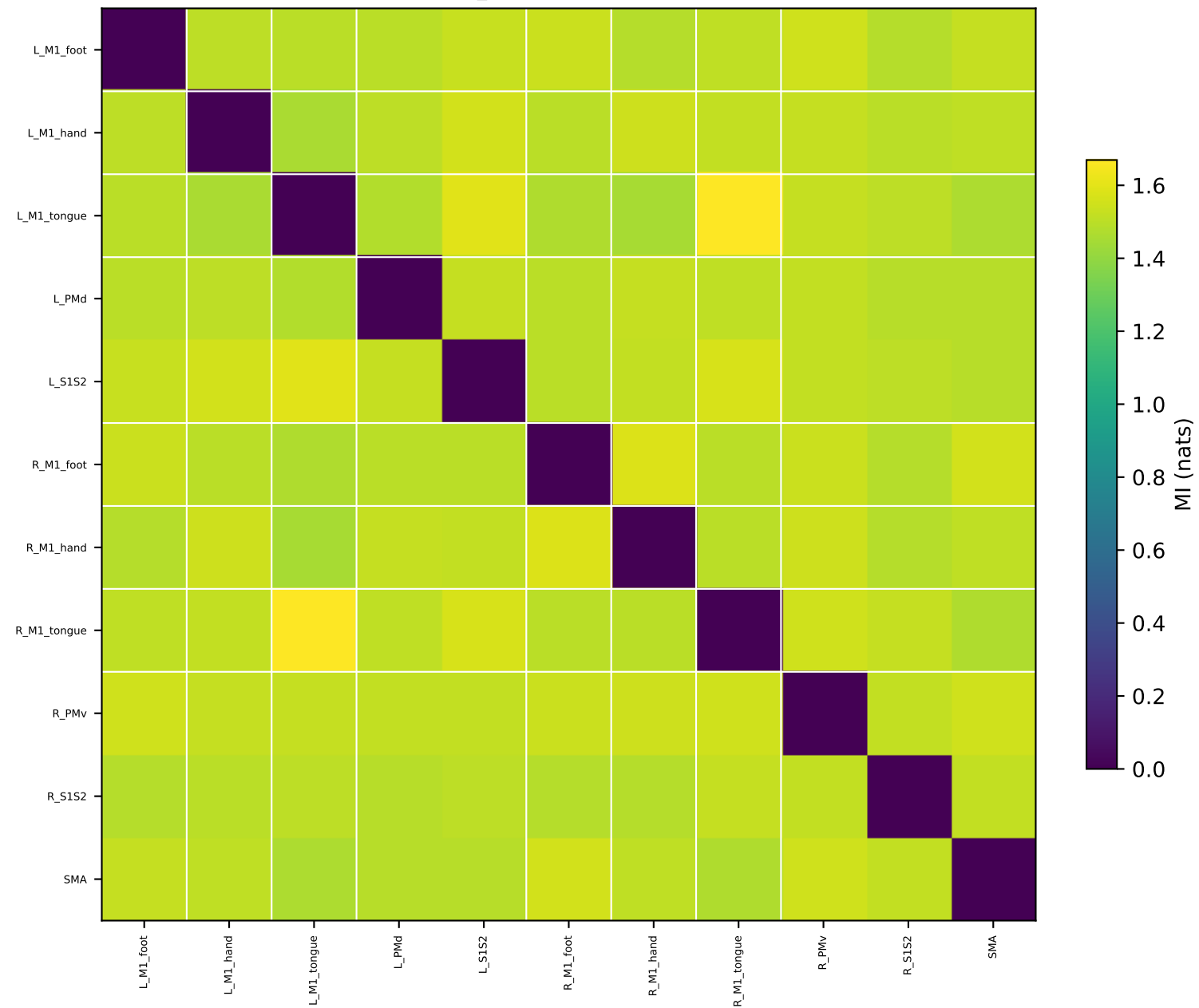
MSC10_func08 — GCSS Motor MI
