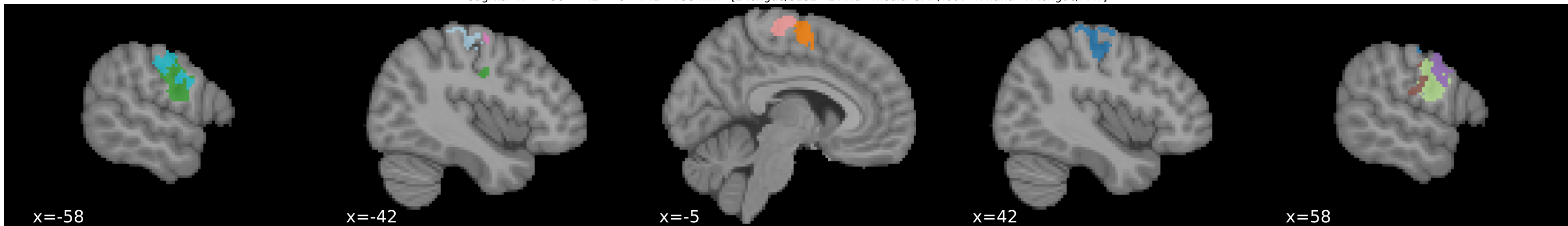
Sagittal x = -58 \cdot -42 \cdot -5 \cdot +42 \cdot +58 mm [L tongue/S1S2 · L PMd · medial SMA/foot · R hand · R tongue/PMv]
