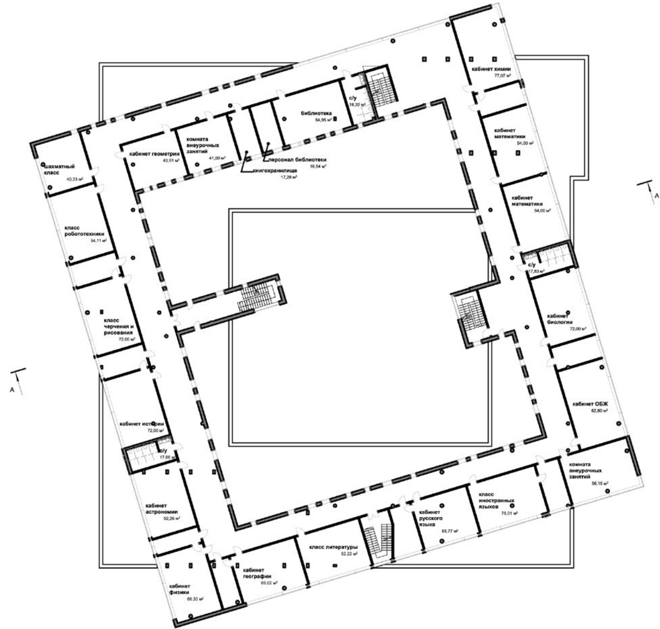
План 3-го этажа
