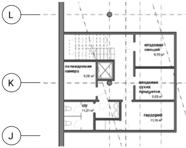
План подвального этажа
