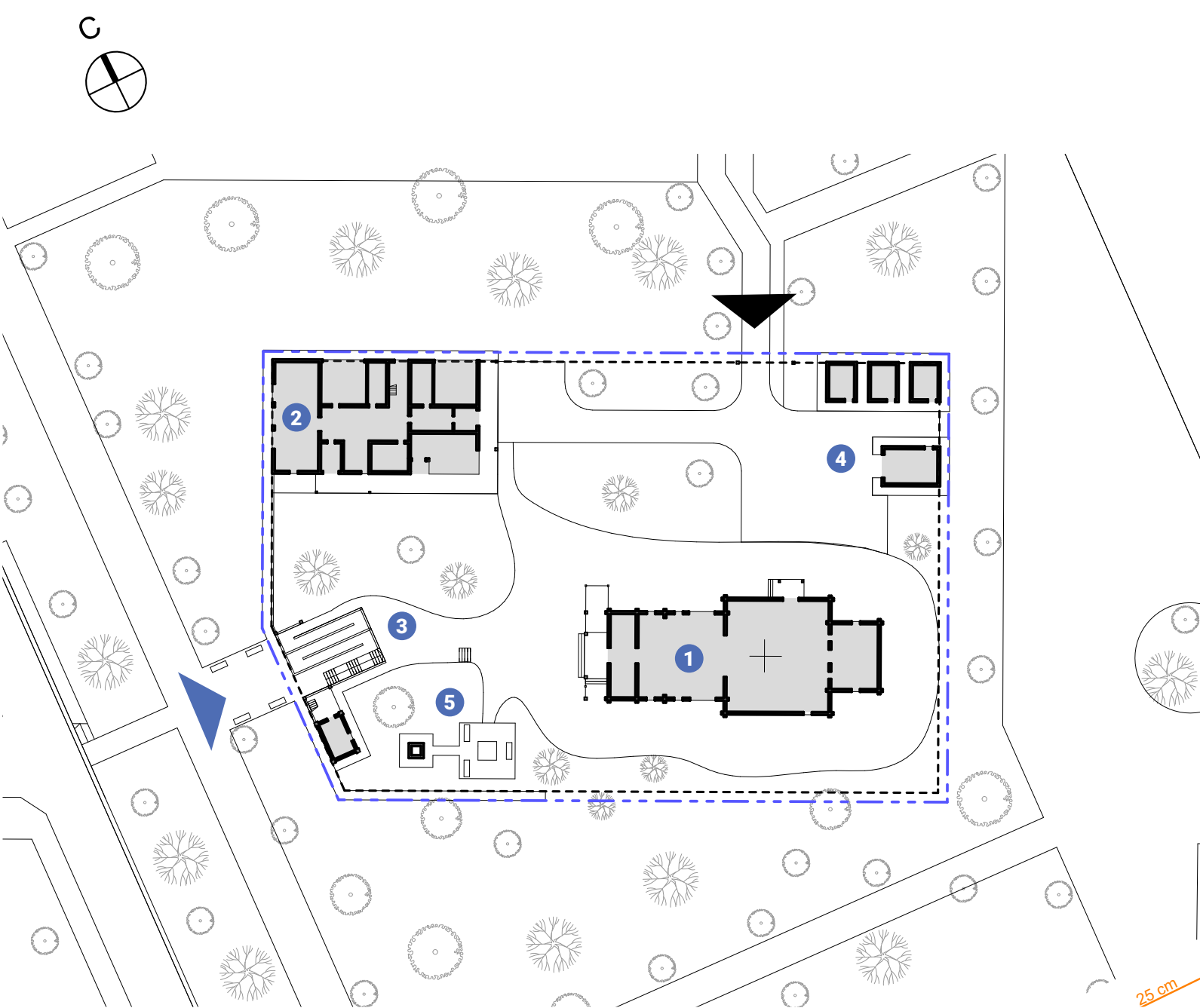
Генеральный план
