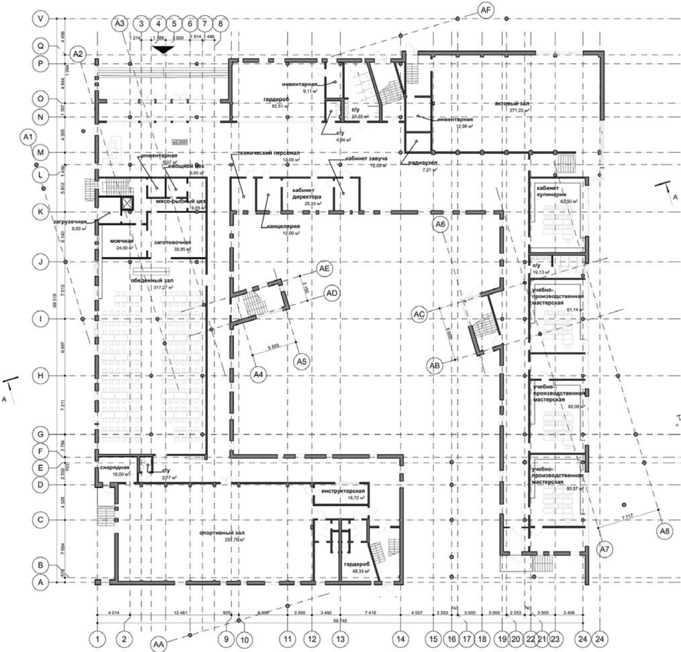
План 1-го этажа
