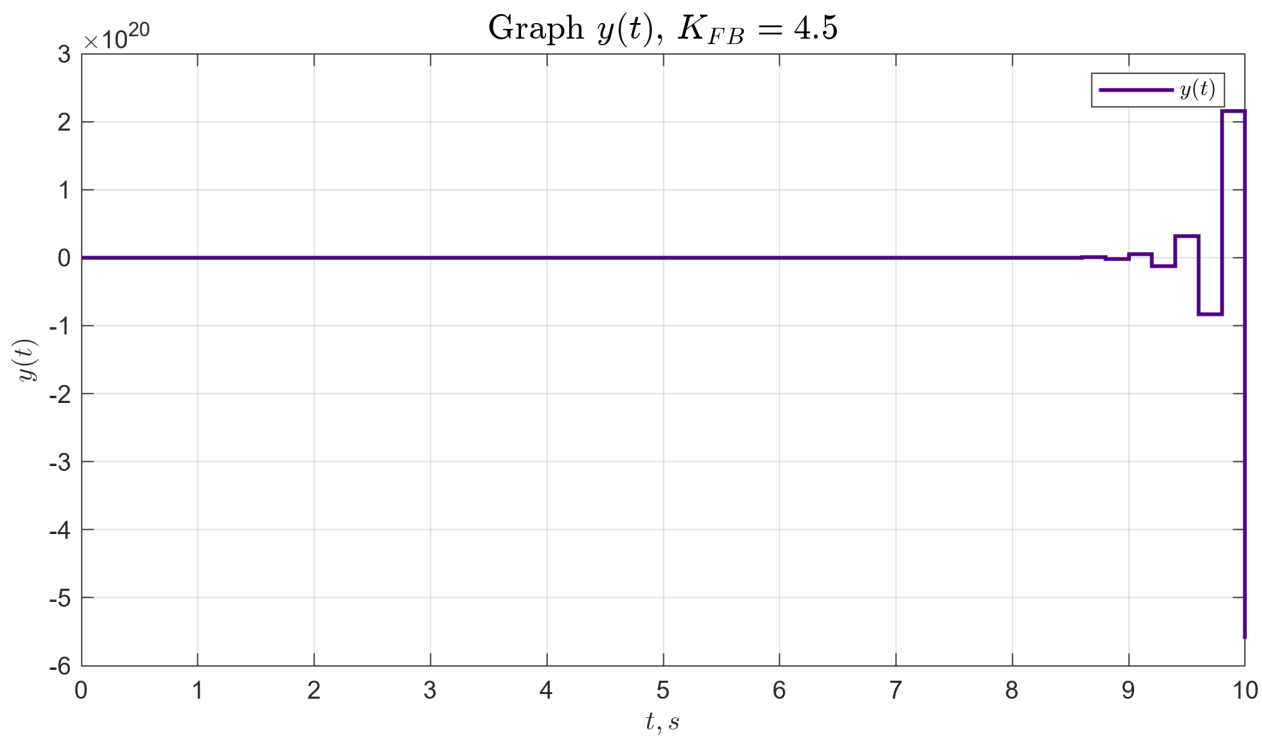
Рисунок 11 — График переходного процесса при K_{FB} = 4.5
