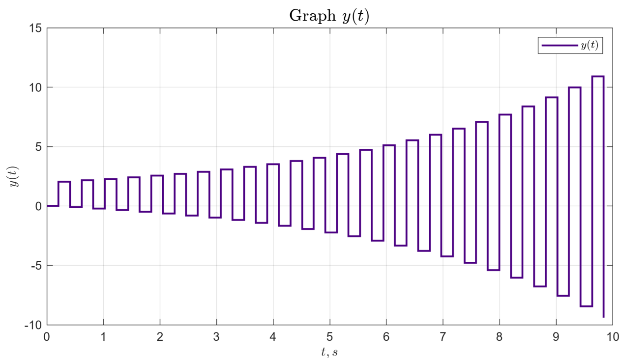
Рисунок 4 — График переходного процесса при K_{FB} = 2.5 и T = 0.205 с.
