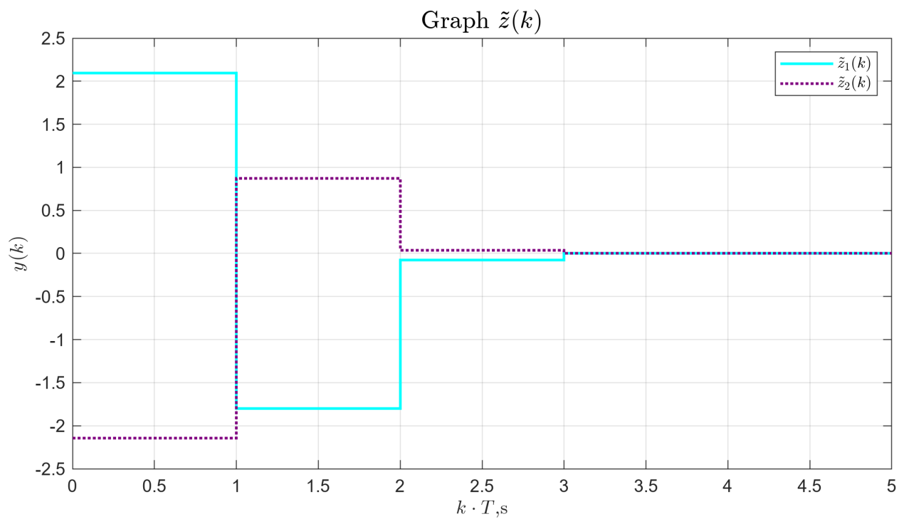
Рисунок 14 — График невязки наблюдателя \tilde{z}(k) .
