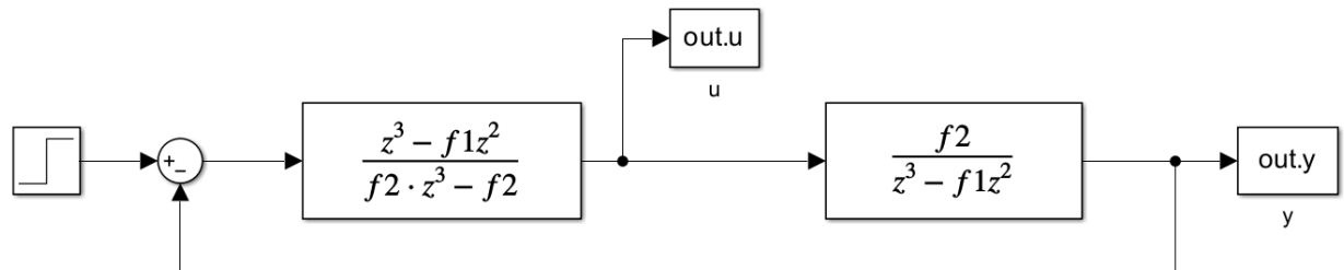
Рисунок 1 — Схема моделирования замкнутой системы с аperiодическим регулятором.
