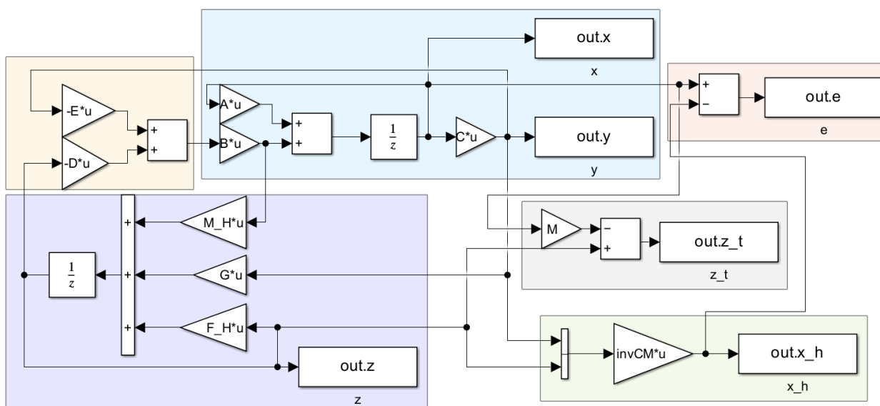
Рисунок 10 — Схема моделирования замкнутой системы из первой главы с устройством оценки пониженной размерности.
