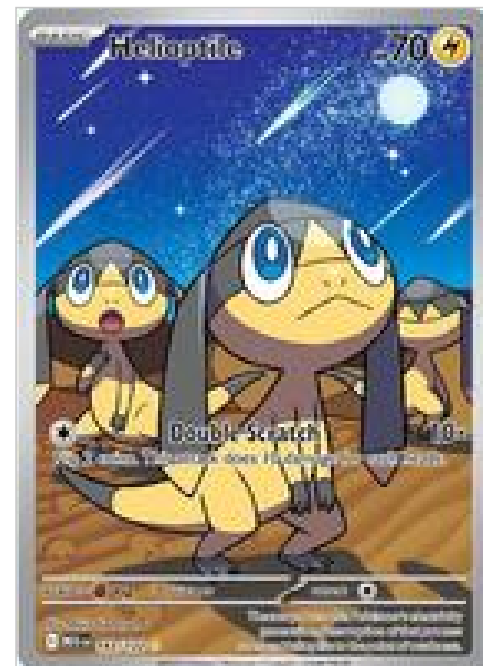
Helioptile - 143/132
