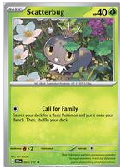
Scatterbug - 005/191
