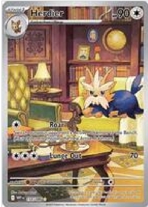
Herdier - 155/086
