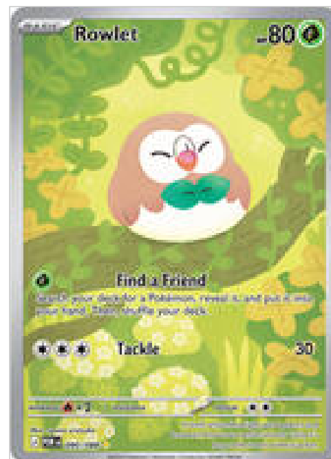
Rowlet - 090/088
