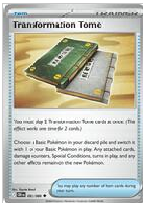
Transformation Tome - 083/086
