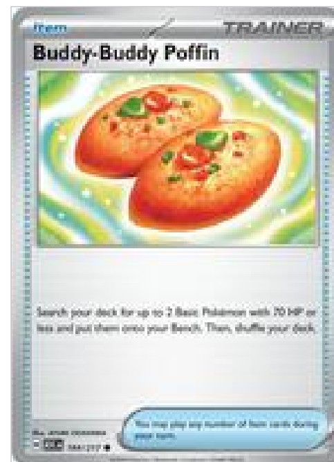
Buddy-Buddy Poffin - 184/217
