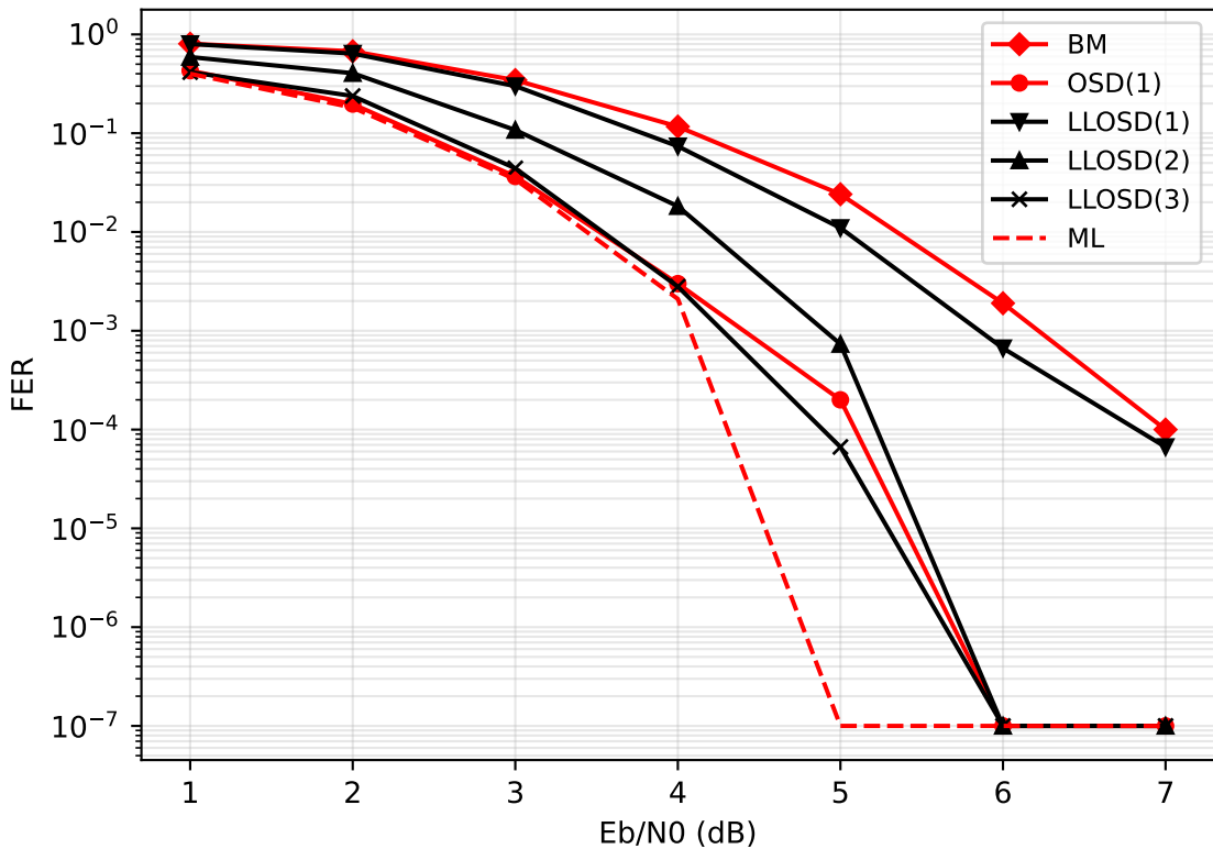
Fig. 4: (63, 45) BCH code
