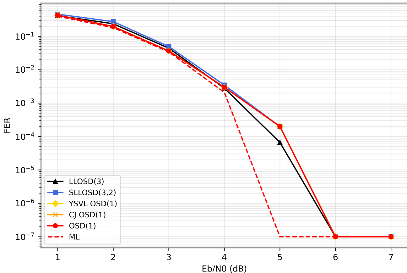
Fig. 5: (63, 45) BCH — LLOSD/SLLOSD/YSVL/CJ vs OSD/ML
