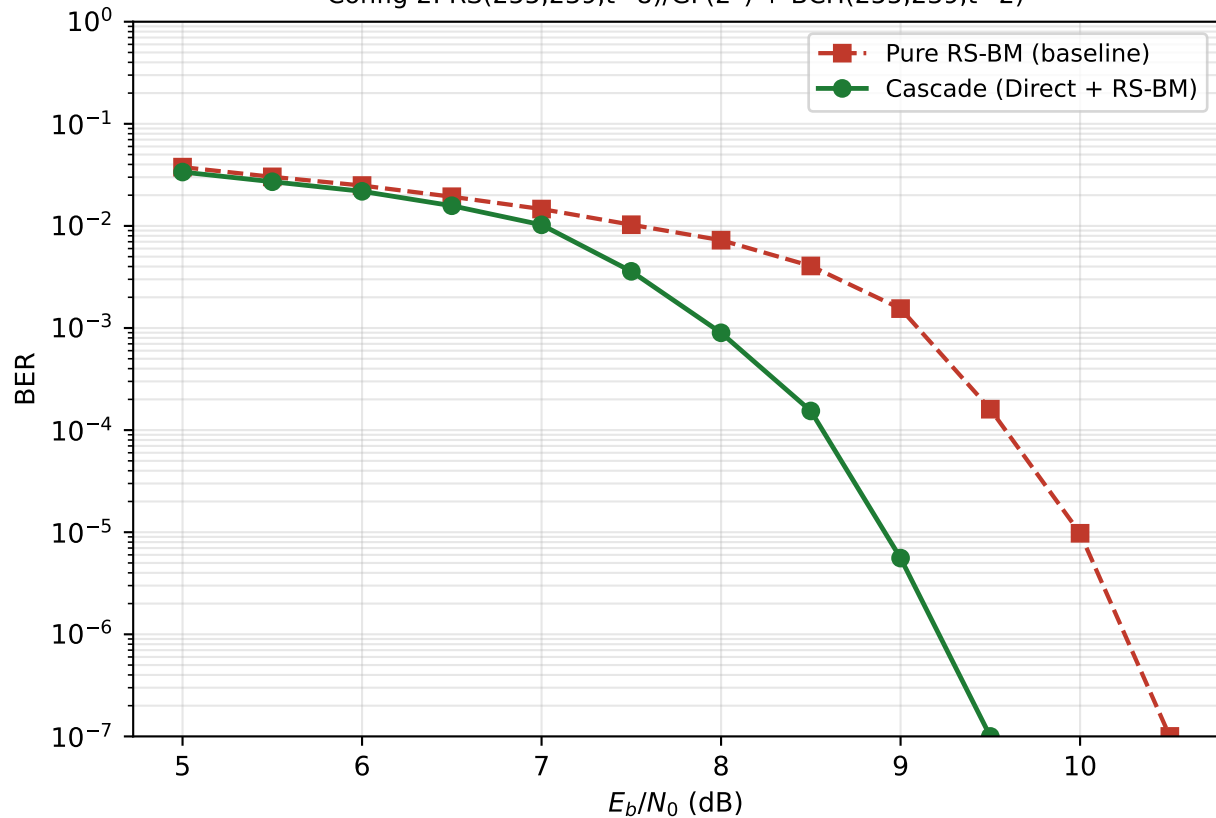
Config 2: RS(255,239,t=8)/GF(2 8 ) + BCH(255,239,t=2)
