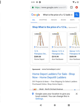
test.png
