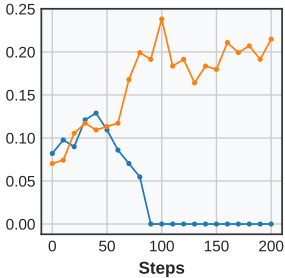
Sokoban
