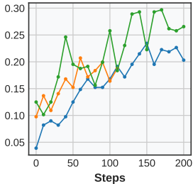
Sokoban
