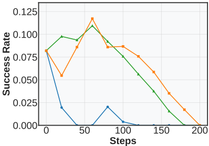
Sokoban (PPO)
