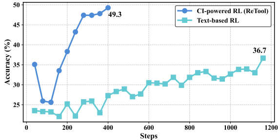
AIME 2025
