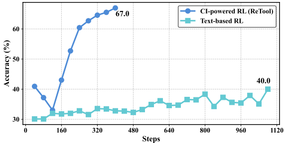
AIME 2024
