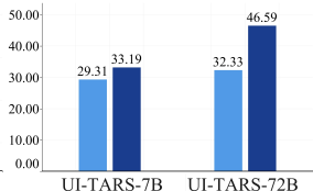
AndroidWorld(Bo1)
