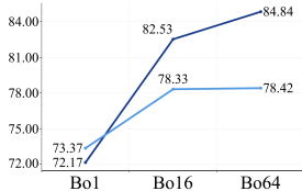
AndroidControl
