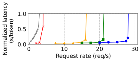
(d) OPT-13B, 1 GPU, Alpaca
