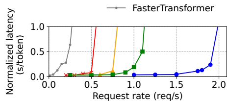
(a) OPT-13B, 1 GPU, ShareGPT
