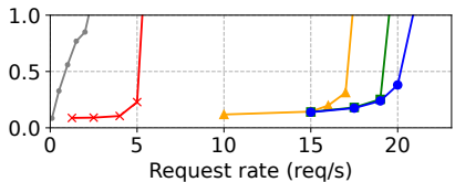
(f) OPT-175B, 8 GPUs, Alpaca
