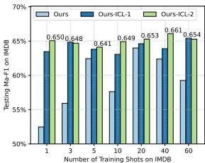
(a) IMDB-IMDB@Mi-F1, Ma-F1
