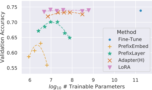
WikiSQL
