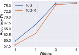
WebQSP
