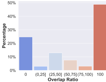
WebQSP
