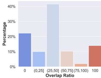
CWQ
