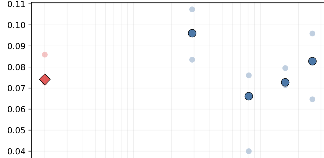
Absolute-ACF MAE, lags 1-4
