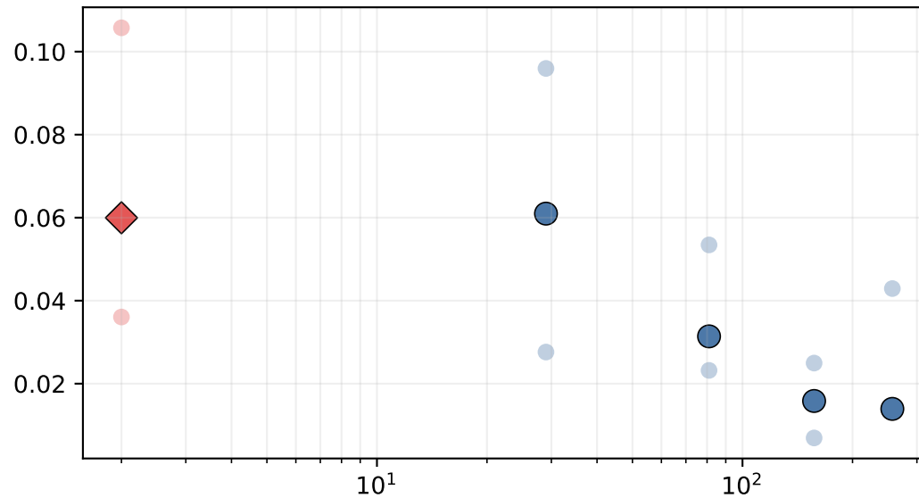
Raw-ACF MAE, lags 1-4
