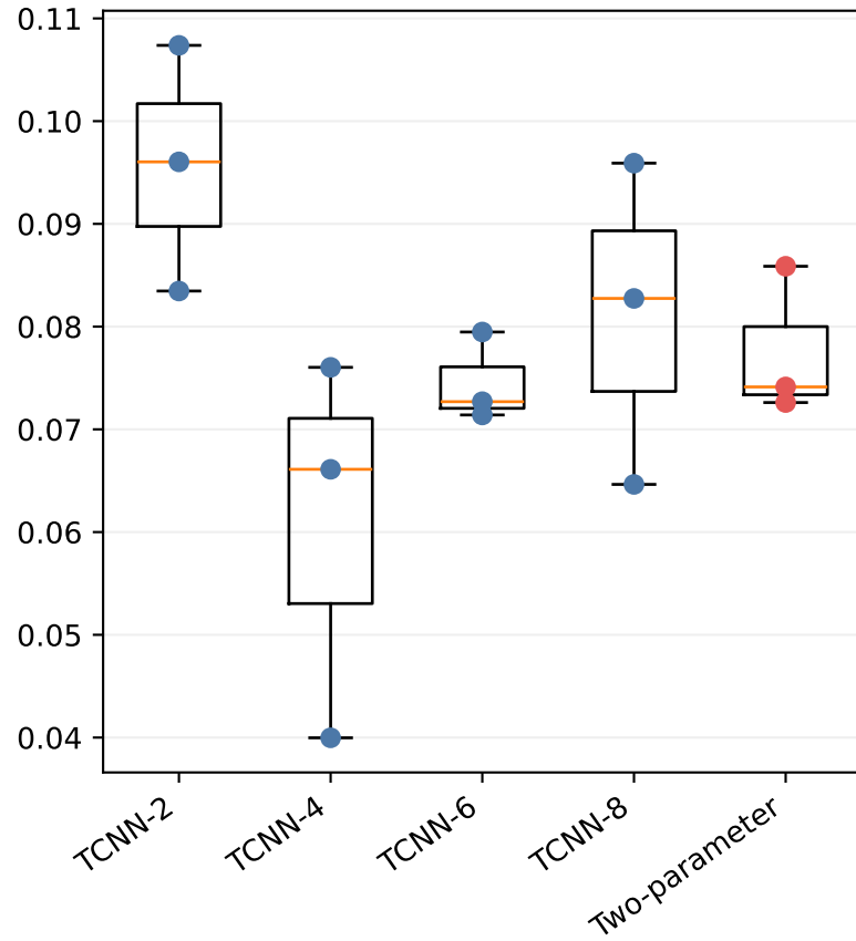
Absolute-ACF MAE
