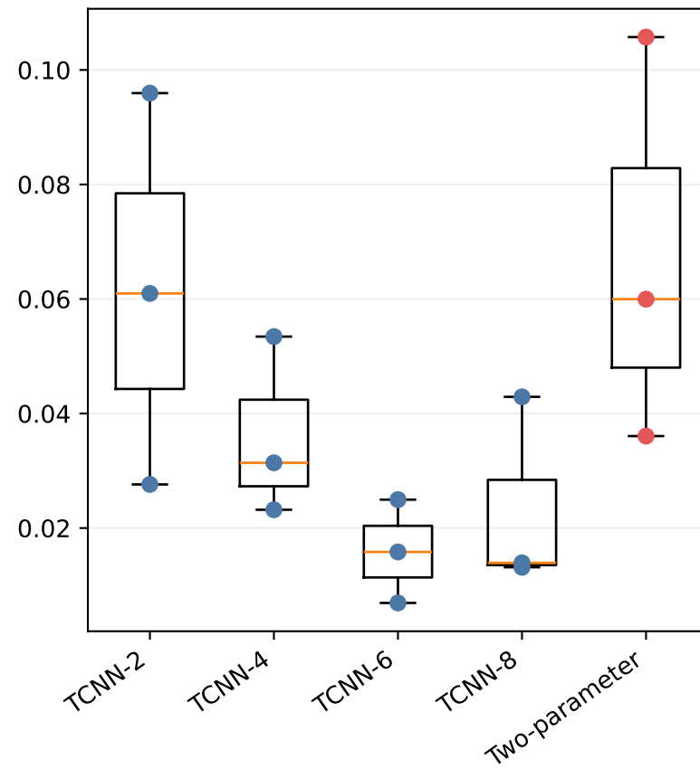
Raw-ACF MAE
