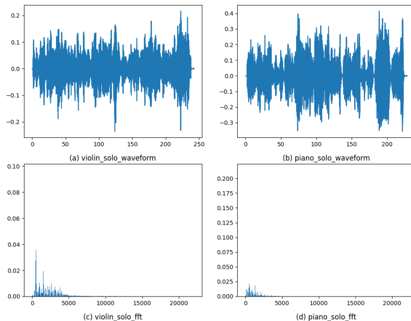
圖 3.4: 兩種資料的波型圖與經過 FFT 轉換後的頻譜圖：(a) 小提琴波型圖、(b) 鋼琴波型圖、(c) 小提琴 FFT 頻譜圖、(d) 鋼琴 FFT 頻譜圖
