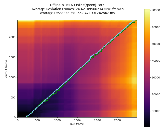
(c) 系統與 DTW 離線追蹤比較圖
