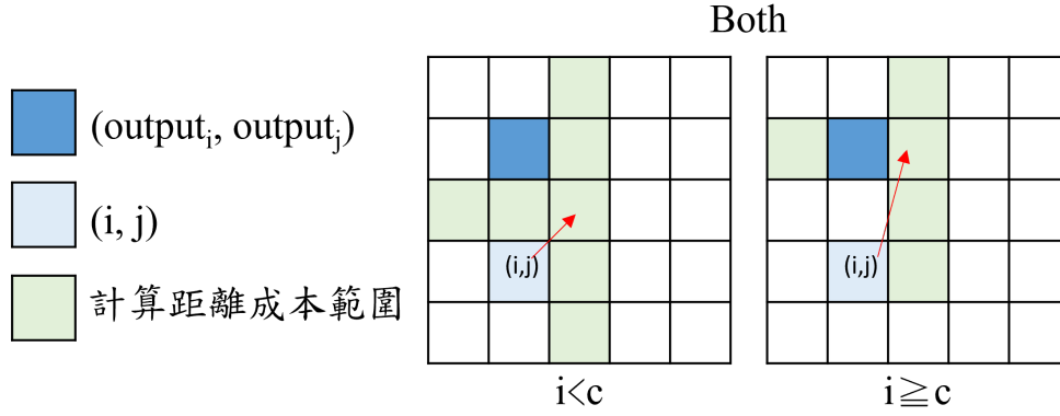
圖 3.12: 改動後 ODTW 決定計算方向示意圖, c = 3
