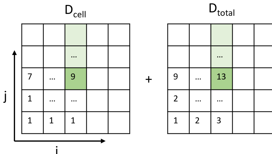
圖 3.10: 改動後 ODTW 計算輸出對齊點範圍示意圖
