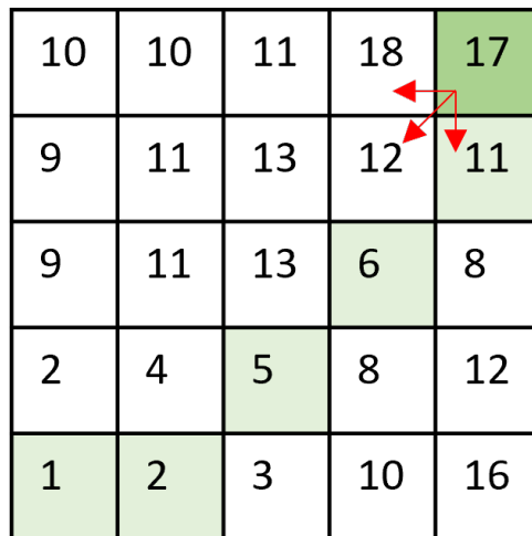
圖 3.6: DTW 累積距離成本矩陣回溯路徑示意圖
