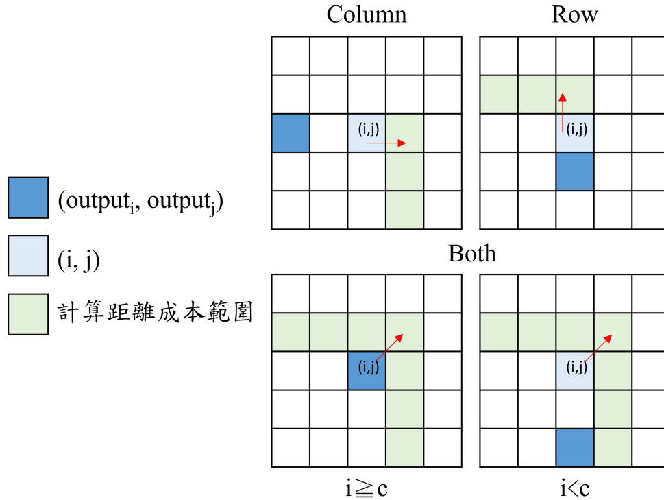
圖 3.11: 傳統 ODTW 決定計算方向示意圖, c = 3
