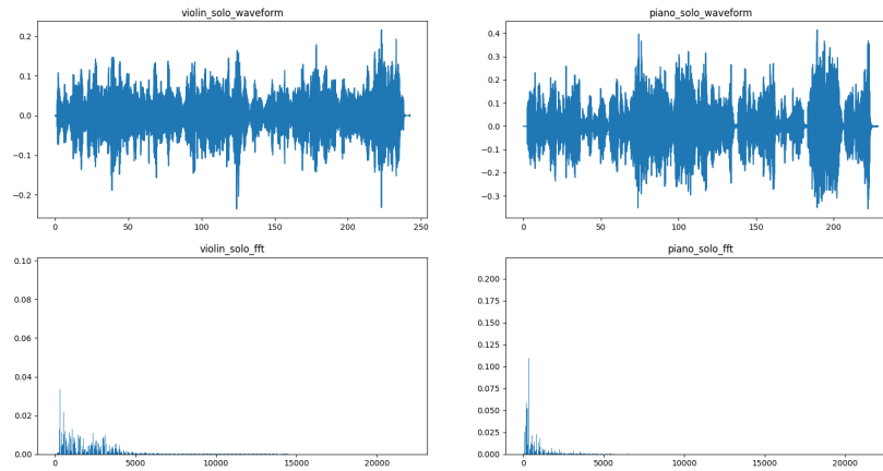
圖 3.3: 兩種資料的波形圖 (上) 與經過 FFT 轉換後的 F_{band} 圖 (下)
