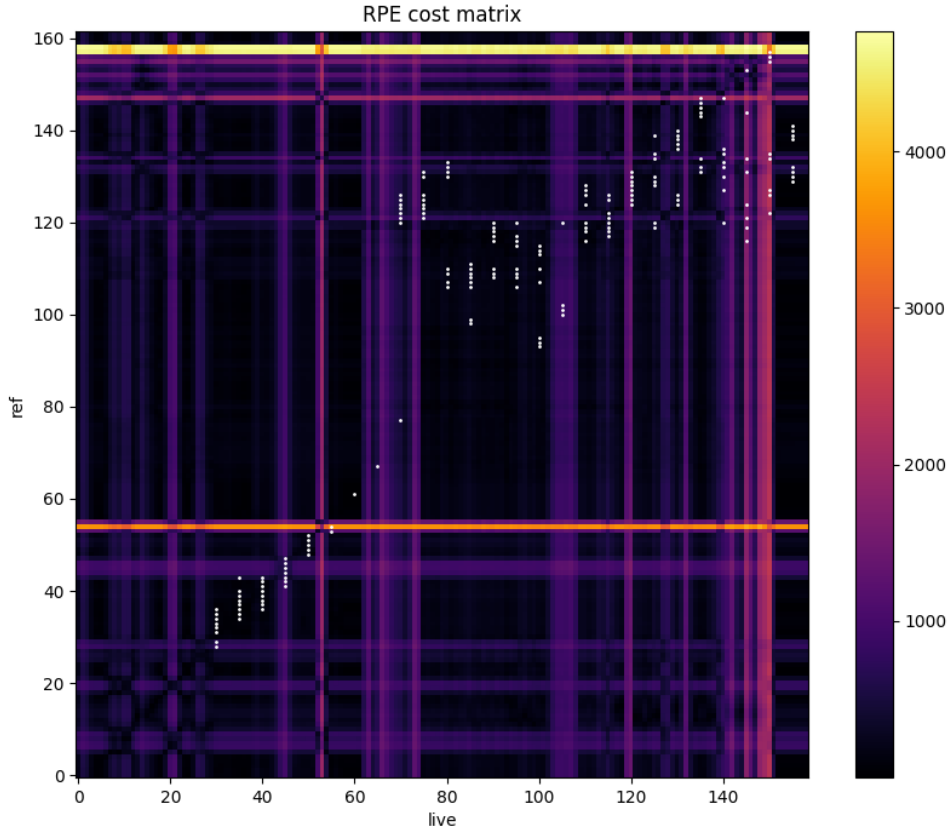
圖 3.16: 粗略位置估計器的輸出位置
