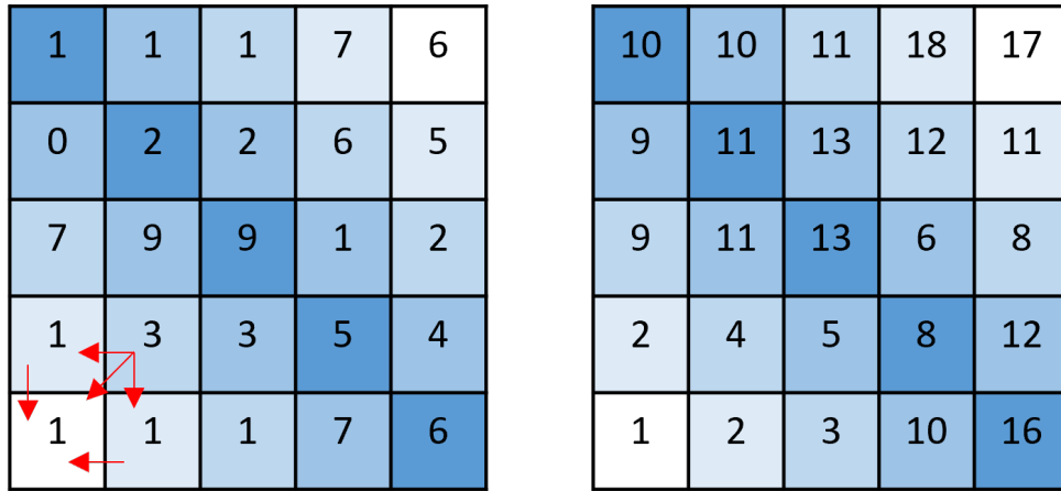
圖 3.5: DTW 累積距離成本矩陣計算示意圖
