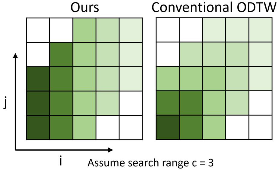
圖 3.8: 每次迭帶所計算到的距離成本矩陣格數位置比較
