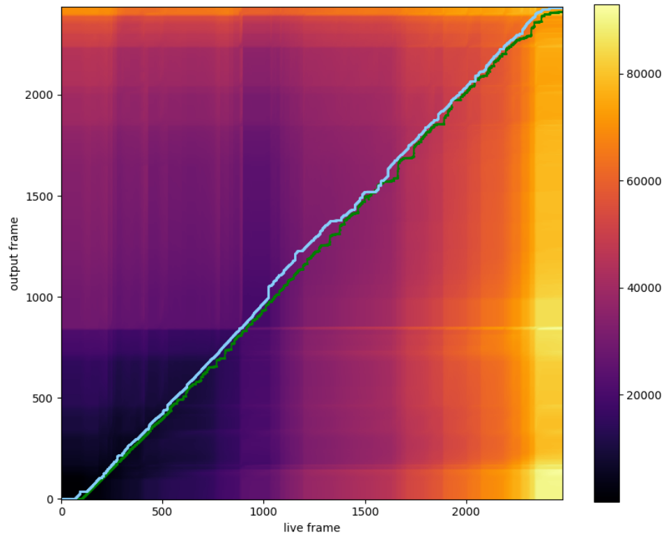
圖 3.18: DTW 與系統的輸出路徑比較圖
