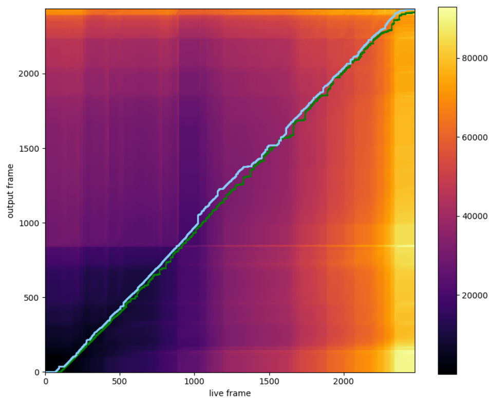
圖 3.19: DTW 與系統的輸出路徑比較圖
