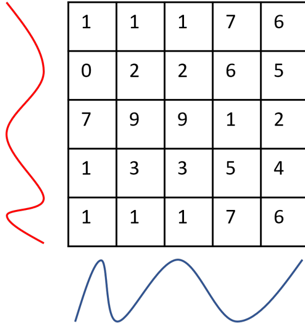
圖 3.5: DTW 單格成本距離矩陣示意圖
