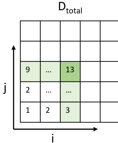
圖 3.10: 傳統 ODTW 計算輸出對齊點範圍示意圖
