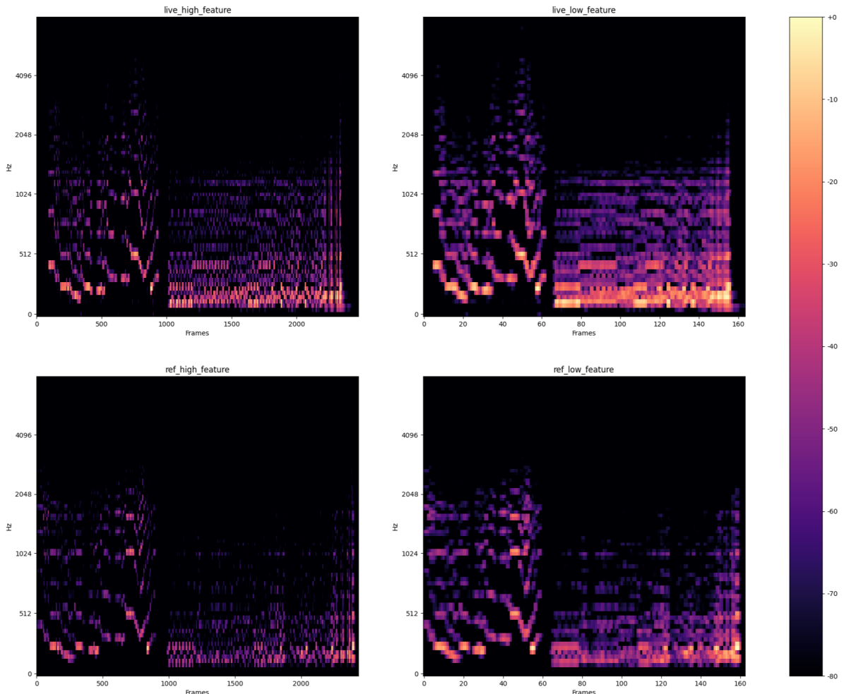
圖 3.15: 上：現場音訊的高 (左) / 低 (右) 解析度特徵圖；下：參考音訊的高 (左) / 低 (右) 解析度特徵圖
