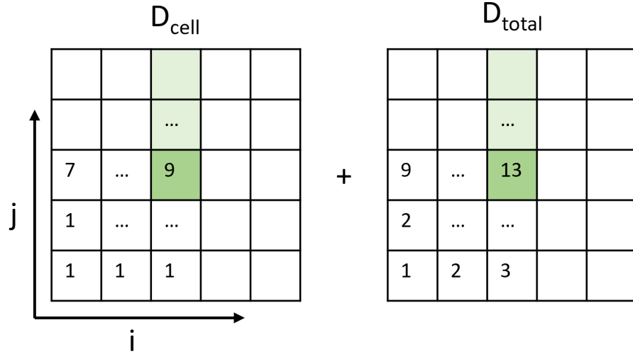
圖 3.11: 改動後 ODTW 計算輸出對齊點範圍示意圖
