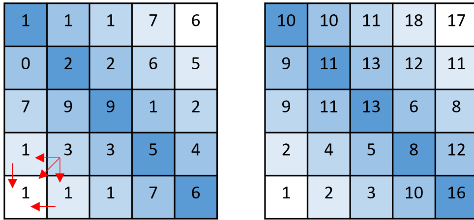
圖 3.6: DTW 累積距離成本矩陣計算示意圖
