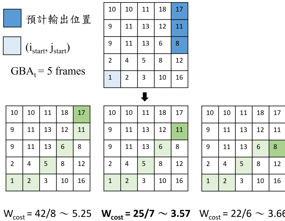
圖 3.14: GBA 計算 W_{cost} 示意圖
