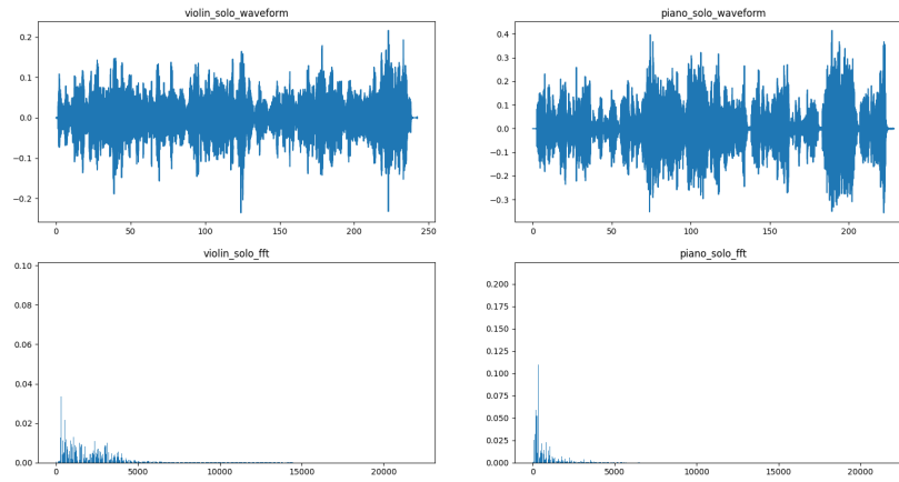
圖 3.3: 兩種資料的波形圖 (上) 與經過 FFT 轉換後的 F_{band} 圖 (下)
