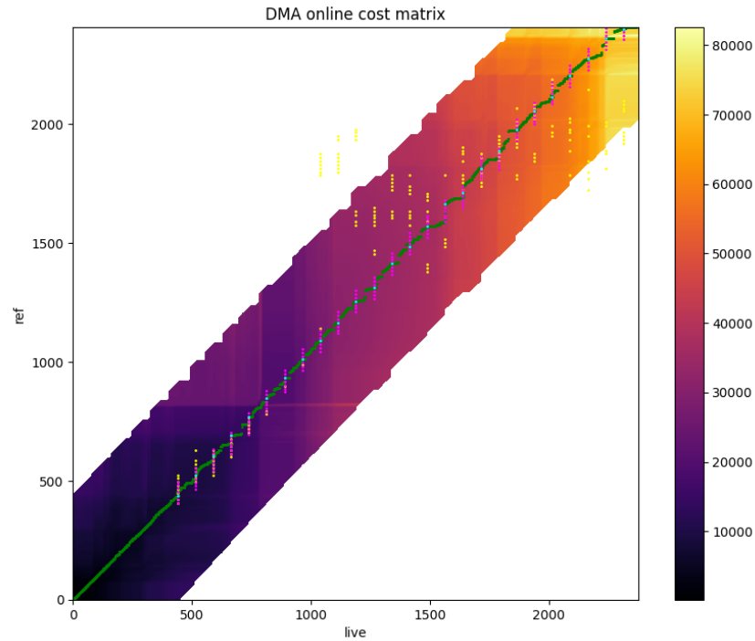
圖 3.18: 追蹤結束後決策決定者輸出的熱力圖與相關元件的輸出點
