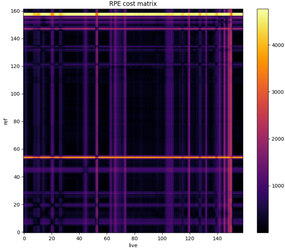
圖 3.16: 粗略位置估計器的距離成本矩陣熱力圖
