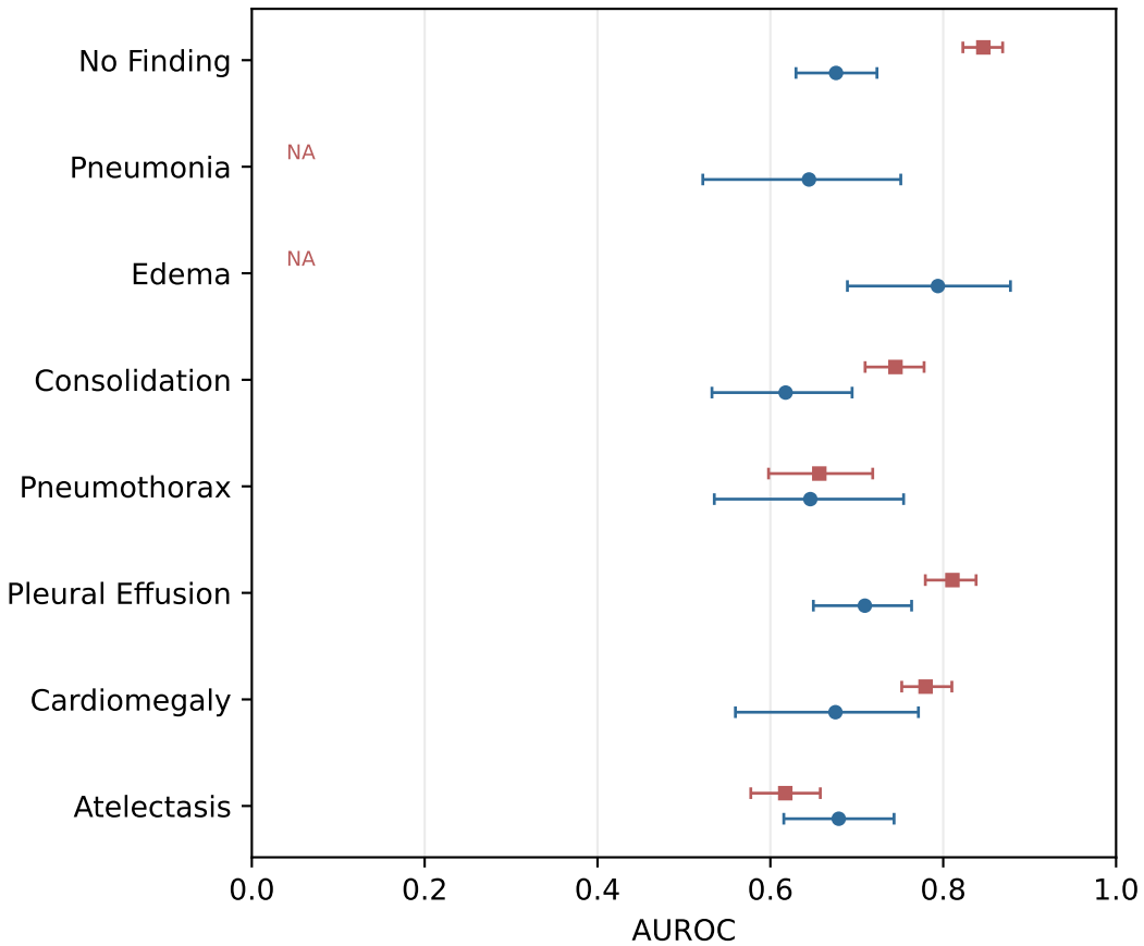
AUROC
