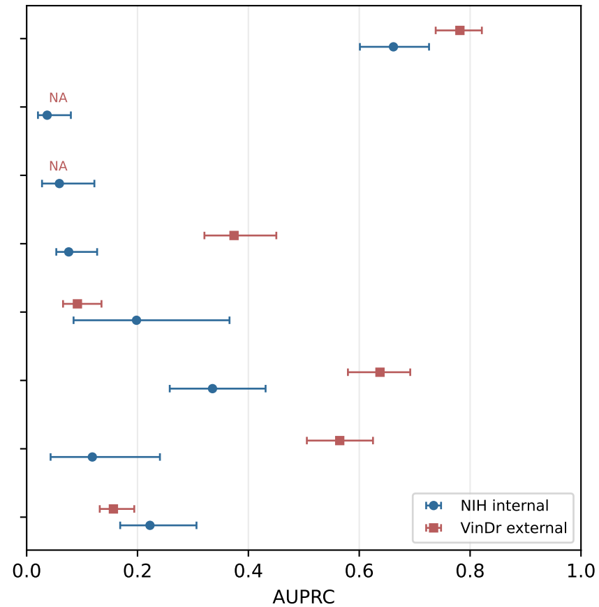
AUPRC
