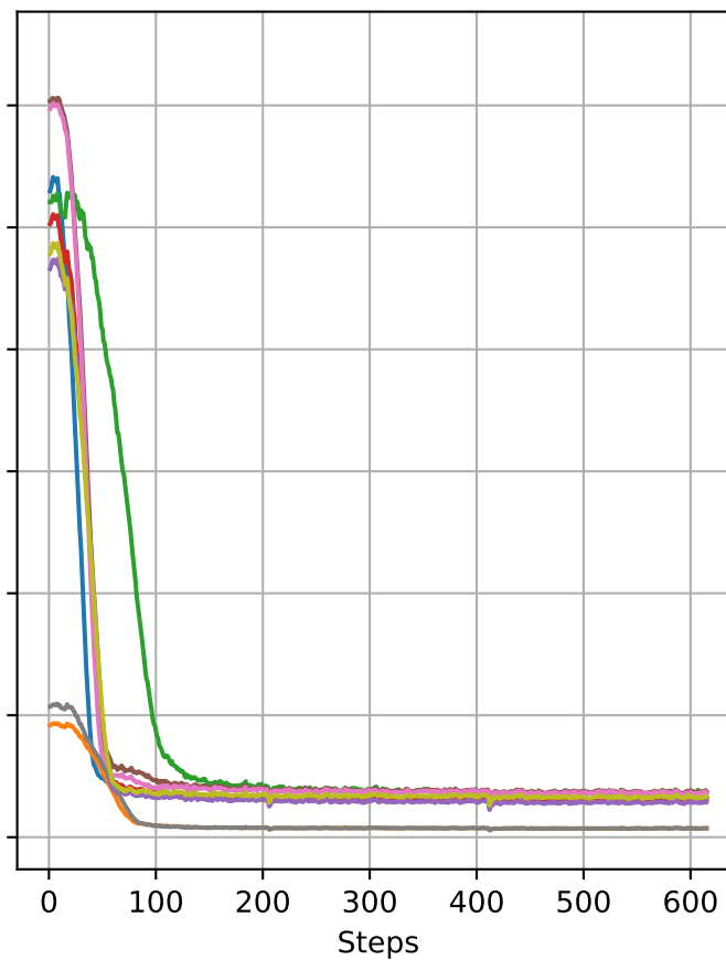
GLOBEM
