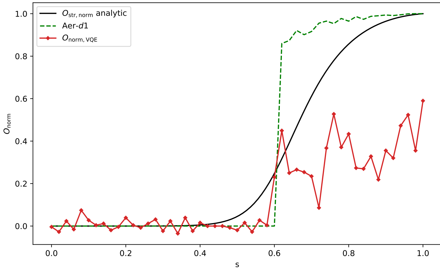
VQE hw+aer sym depth1 delta=-1.0 o
