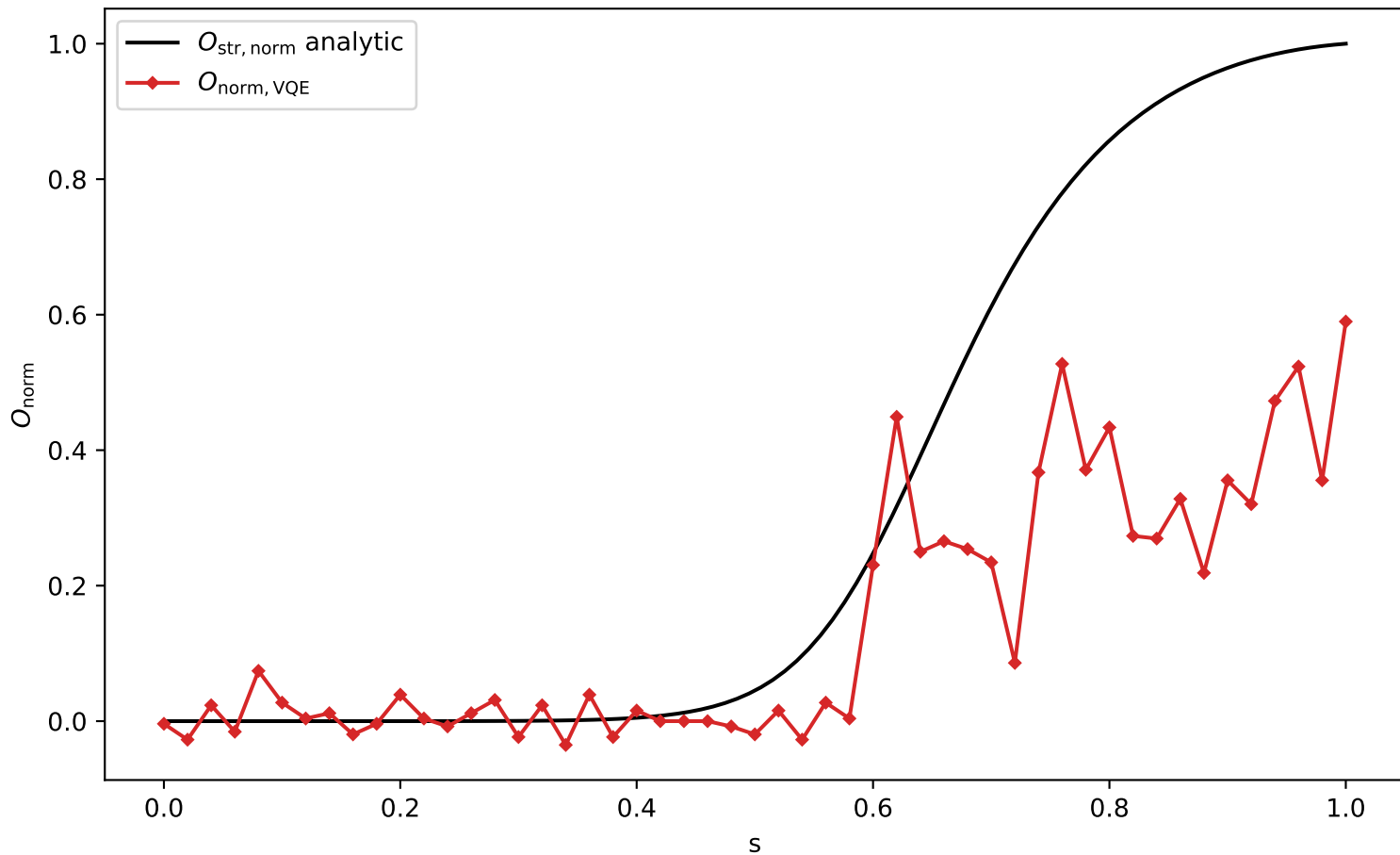
VQE hw sym depth1 delta=-1.0 o
