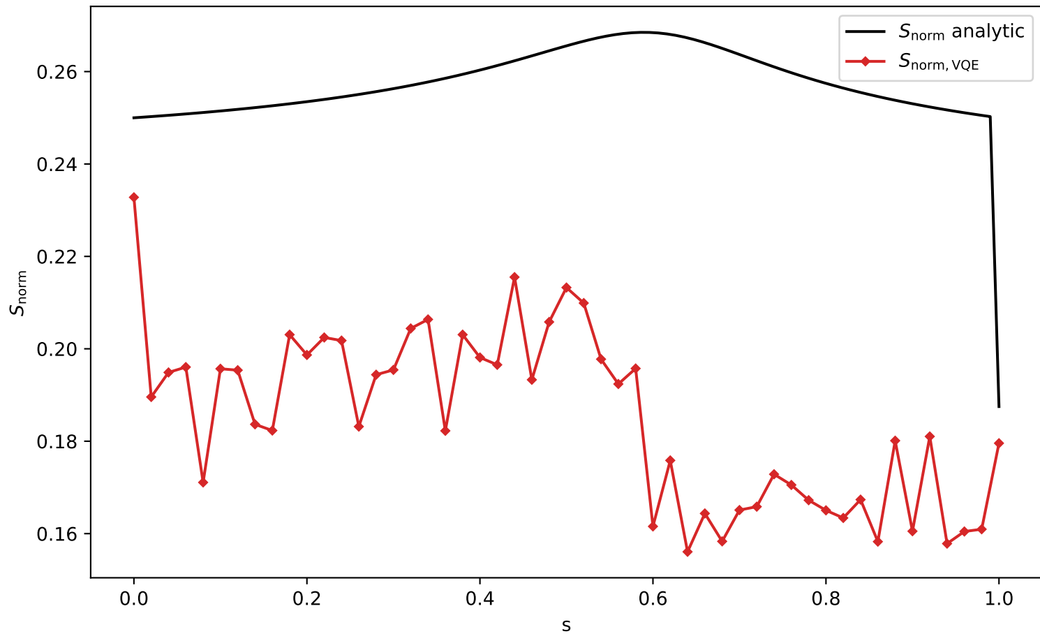
VQE hw sym depth1 delta=-1.0 s
