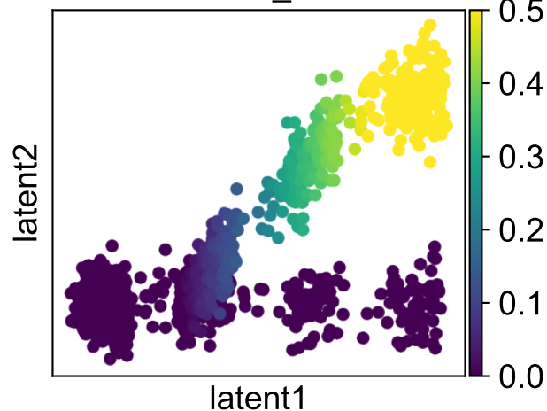
latent_z1
