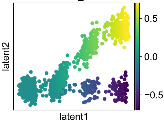
latent_z2
