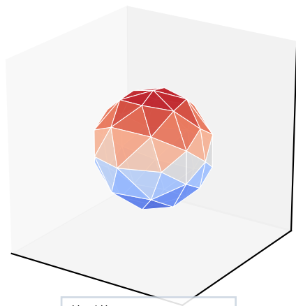
ellipsoid: 球面MDS初期値のみ
