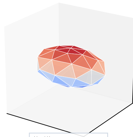
ellipsoid: 辺長実現：0.5%ノイズ
