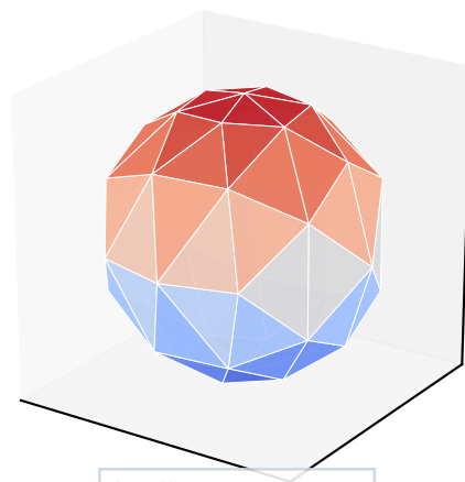
ellipsoid: 辺長実現：無雑音
