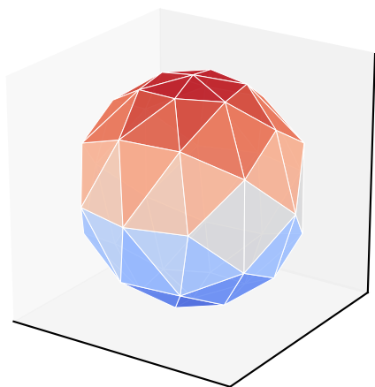
ellipsoid: 正解凸面
