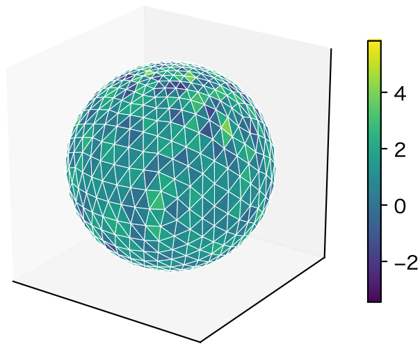
(d) 角度欠損による未平滑化Gauss曲率
