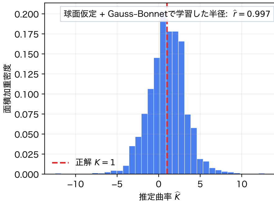
(e) 未平滑化の頂点曲率 (ノイズ感度)
