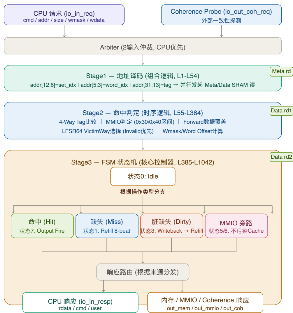
图 3: DUT 数据流图——Cache 模块的 CPU 侧、内存侧与 MMIO 信号通路
