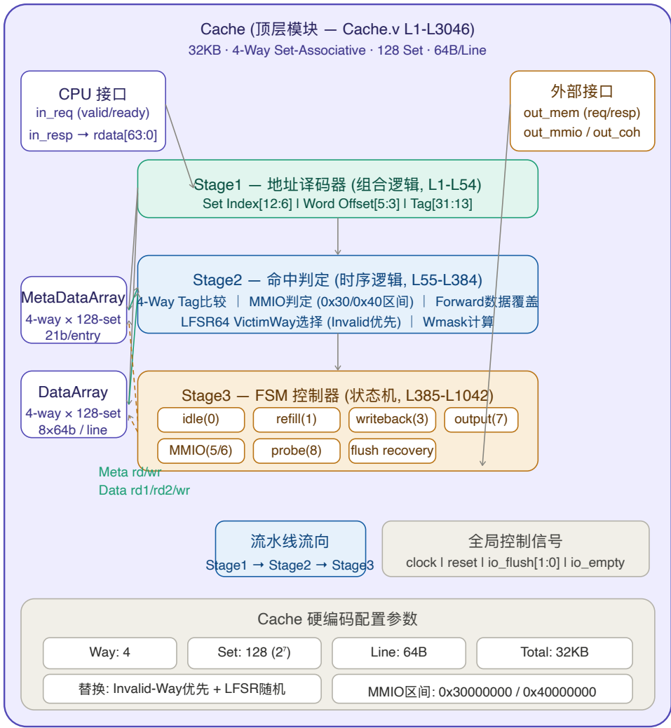
图 4: DUT 层次结构——CacheStage1/2/3 三级流水线及子模块关系
