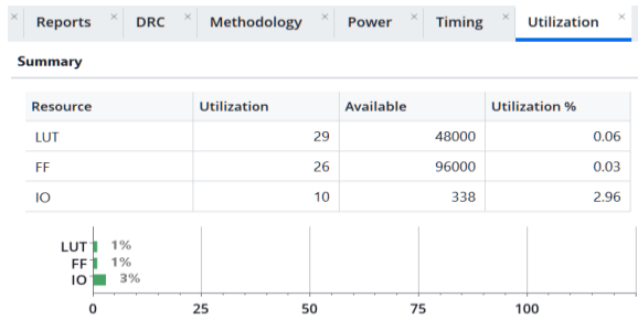
그림 10: 실험 12 클럭 분주기 FPGA 자원 사용량
