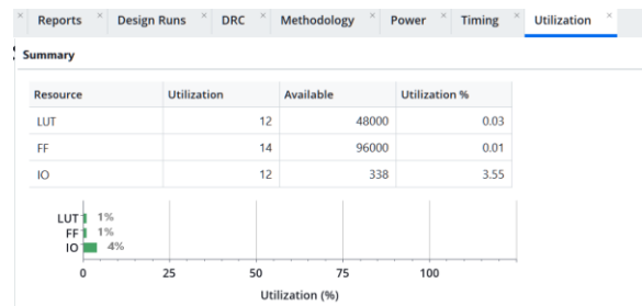
그림 45: 실험 17 Mealy 머신 FPGA 자원 사용량
