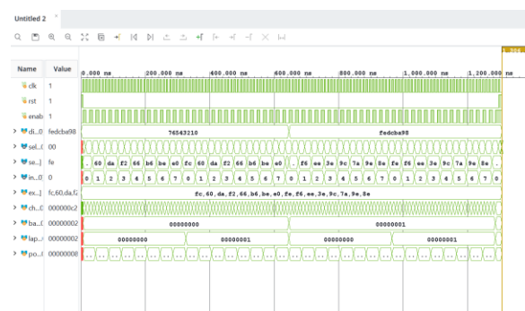
그림 56: 실험 18 입력 조합에 따른 출력 파형
