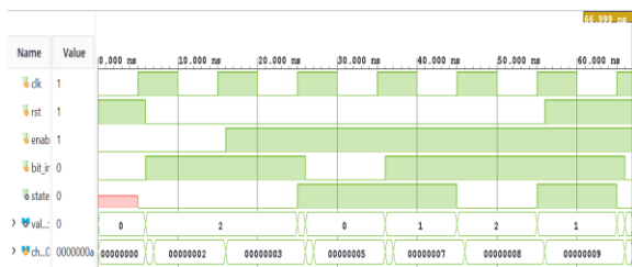
그림 49: 실험 17 입력 조합에 따른 출력 파형
