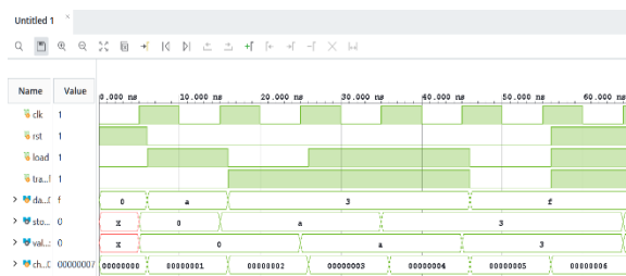
그림 21: 실험 13 입력 조합에 따른 출력 파형
