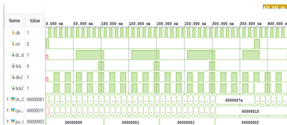
그림 14: 실험 12 입력 조합에 따른 출력 파형
