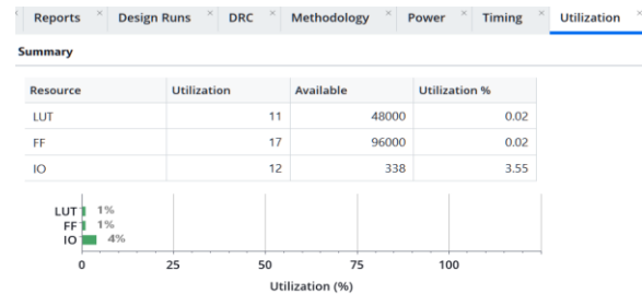
그림 24: 실험 14 shift 레지스터 FPGA 자원 사용량
