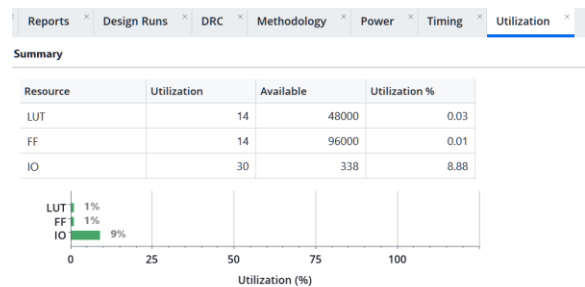
그림 52: 실험 18 7세그먼트 FPGA 자원 사용량
