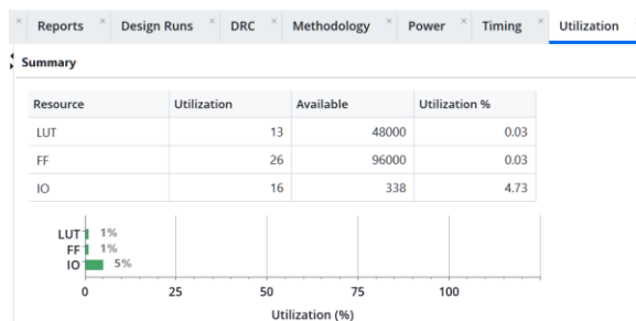
그림 31: 실험 15 PISO FPGA 자원 사용량
