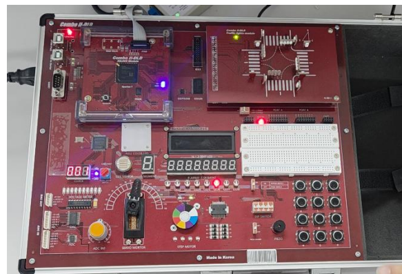
그림 61: 실험 14 FPGA 보드 시연
