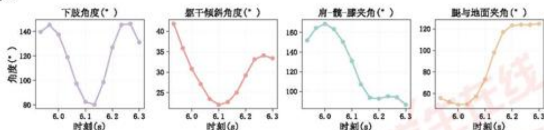
图 17 跳跃阶段四个角度的变化趋势
