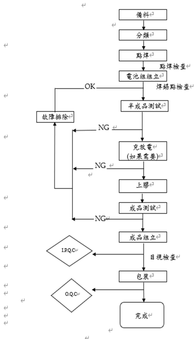
鋰電池製造程序流程圖
