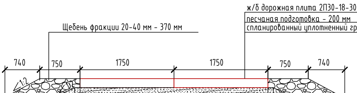
КОНСТРУКЦИЯ ВРЕМЕННЫХ ДОРОГ (ПЛОЩАДОК)
