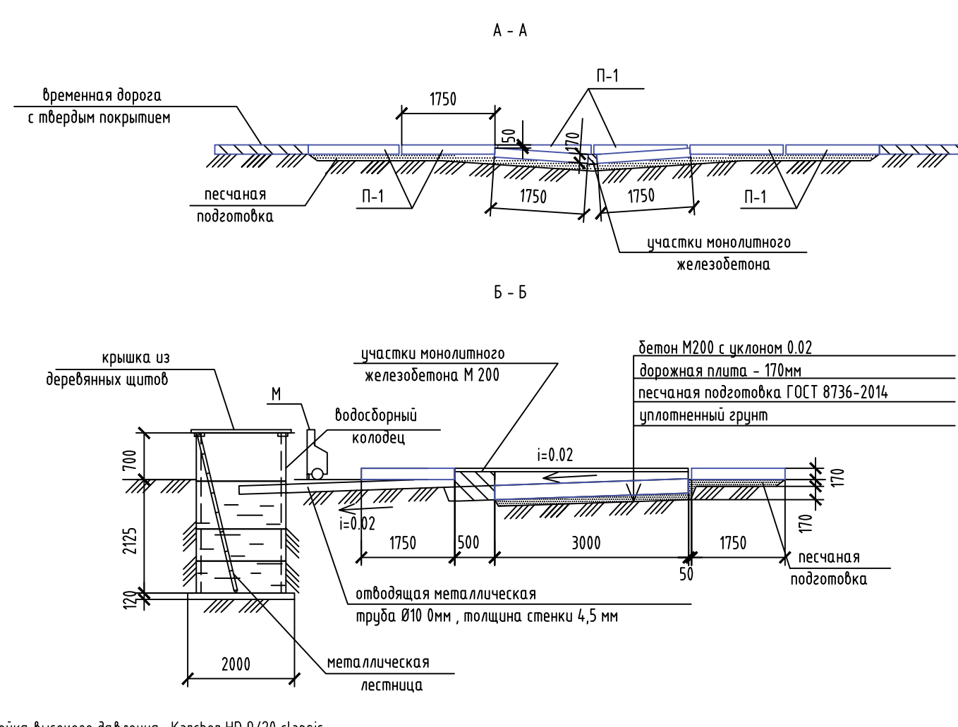
СХЕМА УСТРОЙСТВА ПЛОЩАДКИ ДЛЯ МОЙКИ КОЛЕС АВТОМАШИН
