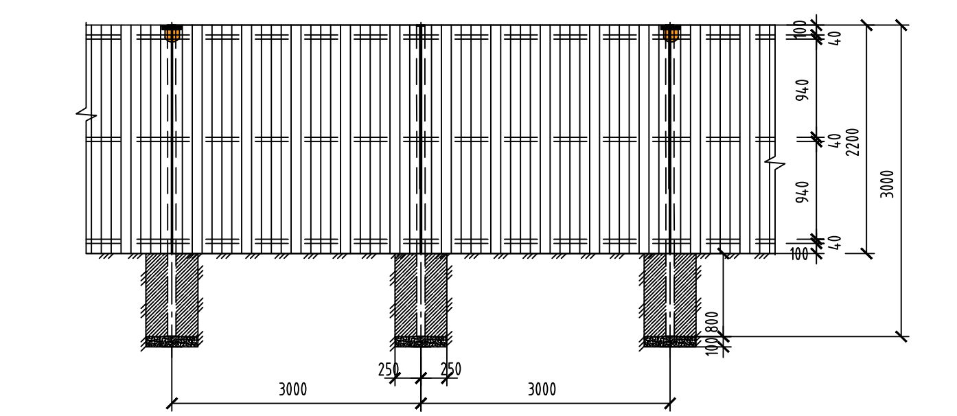
СХЕМА УСТРОЙСТВА ОГРАЖДЕНИЙ СТРОИТЕЛЬНОЙ ПЛОЩАДКИ
