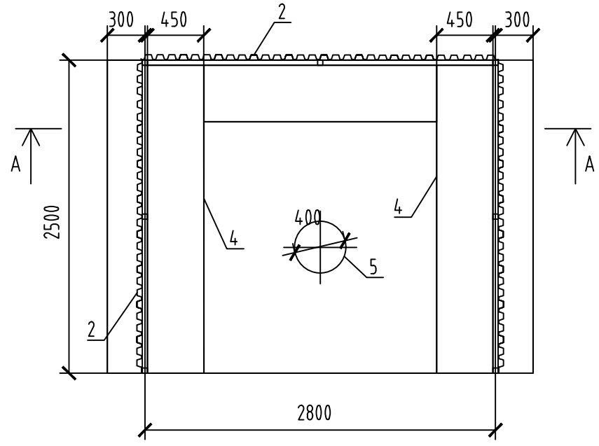
СХЕМА УСТРОЙСТВА МЕСТА ДЛЯ КУРЕНИЯ
