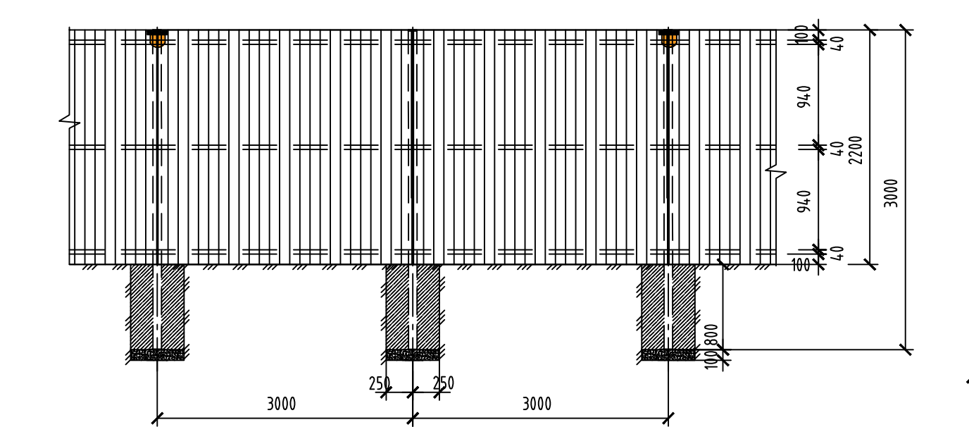
А. Фронтон ограждения строительной площадки без козырька
