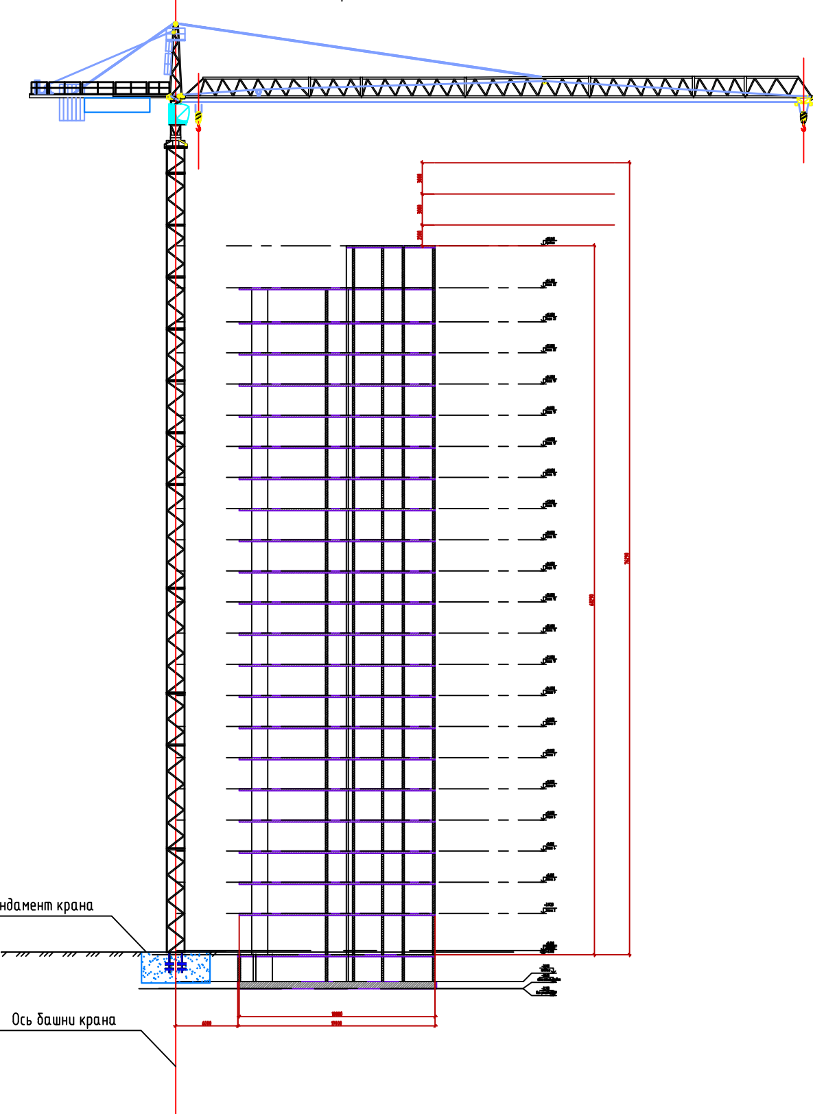
Разрез 1-1
