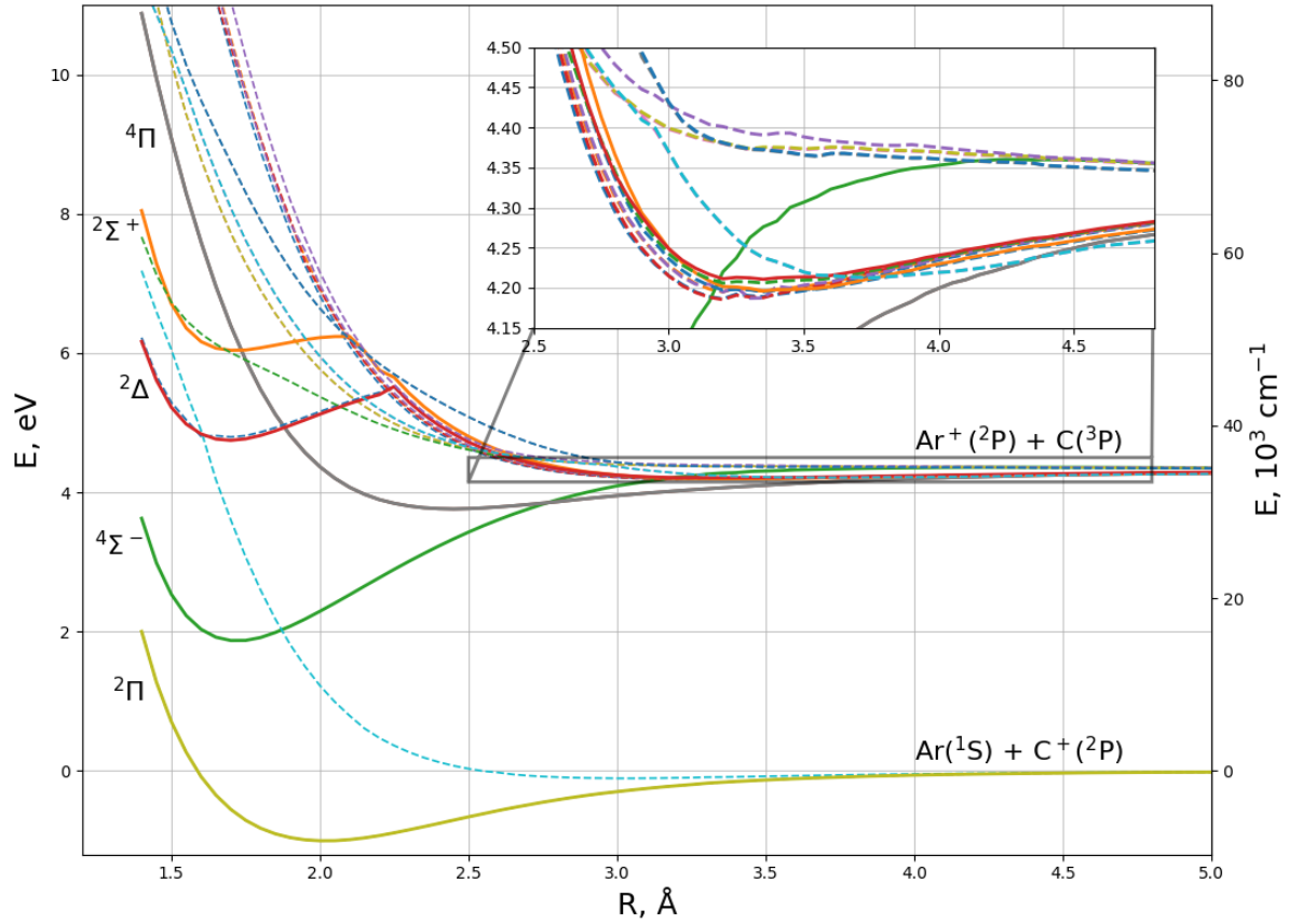
Figure 1: Кривые межатомных потенциалов \text{ArC}^+ без спин-орбитального и спин-спинового расщепления.
