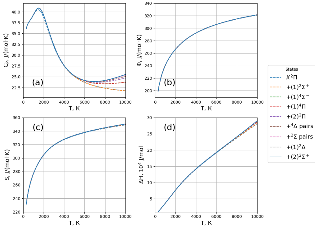
Figure 2: Термодинамические функции \text{ArC}^+ при 298.15 – 10000 K
