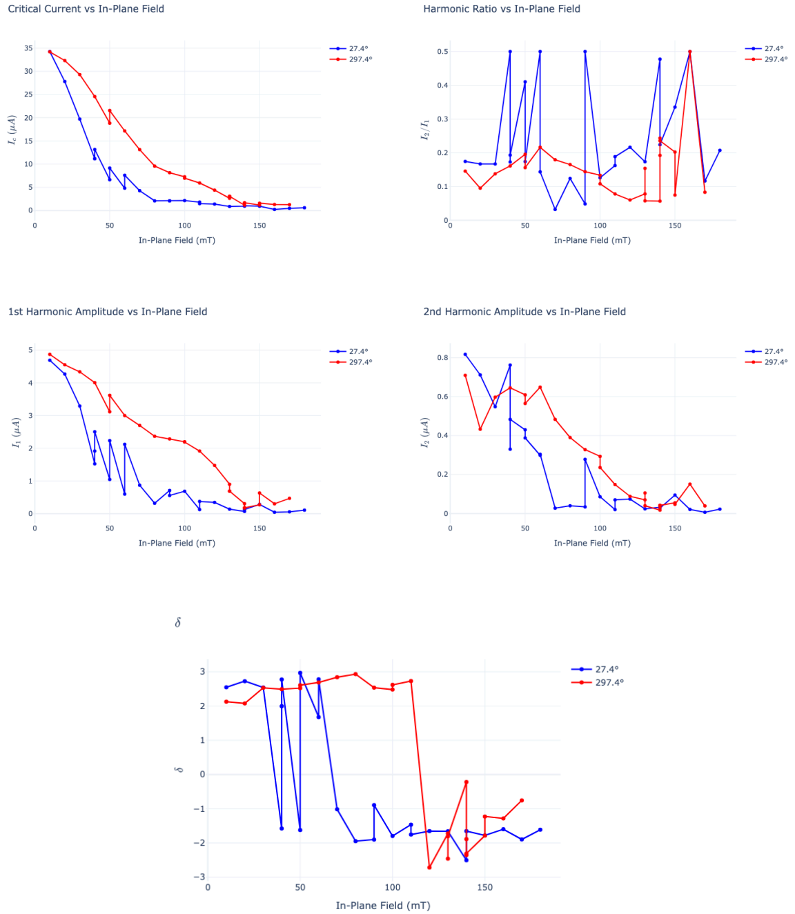
圖 22 Sample 003-2 在特定角度下的參數演化 (27.4° vs 297.4°)。(a) 臨界電流 I_c (b) 諧波比例 \frac{I_2}{I_1} (c) 一階諧波 I_1 (d) 二階諧波 I_2 (e) 相位偏移 \delta 藍色與紅色曲線分別代表
