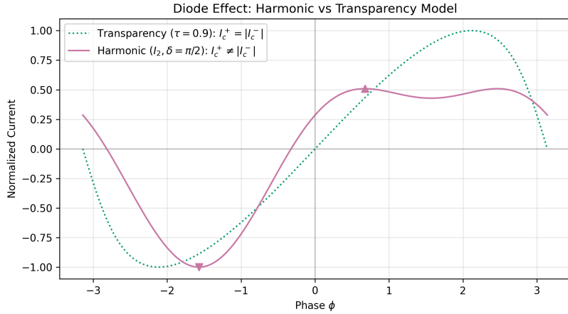
圖 17 透明度模型與谐波模型的比較。標準透明度模型（綠線）雖然能產生偏斜的波形，但仍保持 I_c^+ = |I_c^-| 的對稱性。含有相位偏移的谐波模型（紫線）則能自然描述 I_c^+ \neq |I_c^-| 的約瑟夫森二極體效應。
