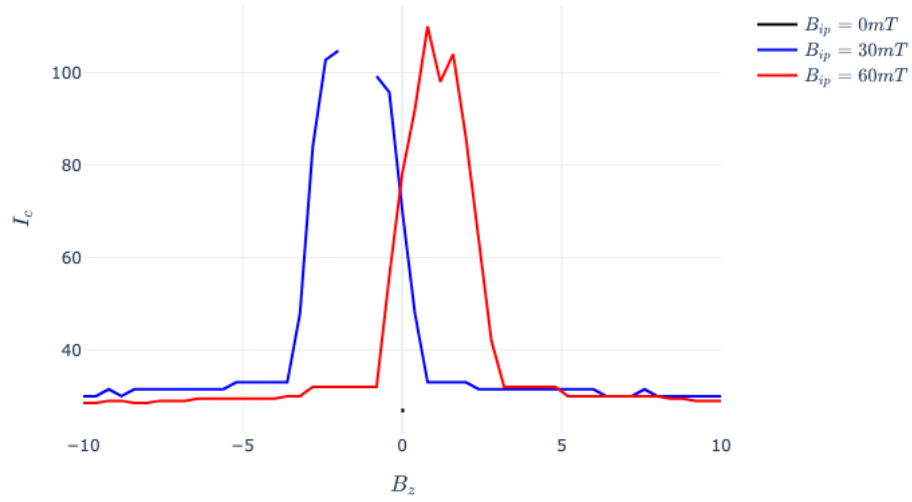
圖 13 面內磁場下夫朗和費圖樣的演化。隨著 B_{\text{in-plane}} 的增加，原本對稱的干涉圖樣逐漸變得不對稱，極小值位置發生偏移，包絡函數形狀也隨之改變。
