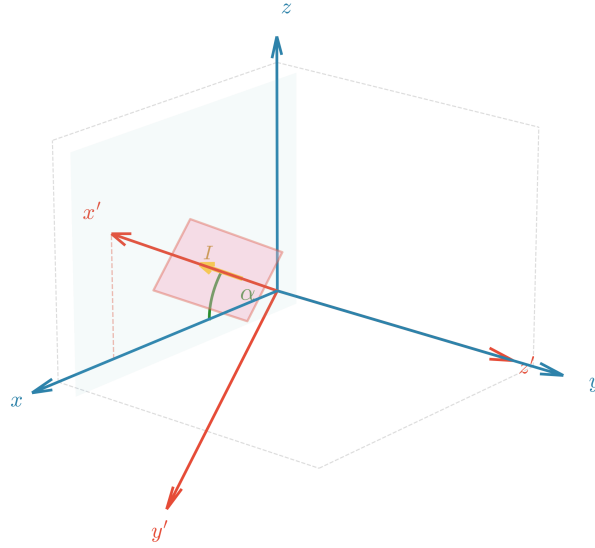
圖 8 實驗室座標系 (X, Y, Z) （藍色）與樣品座標系 (X', Y', Z') （紅色）之幾何關係。樣品平面（粉色矩形）位於 X - Z 平面內，電流方向 X' 與 X 軸夾角為 \alpha 。
