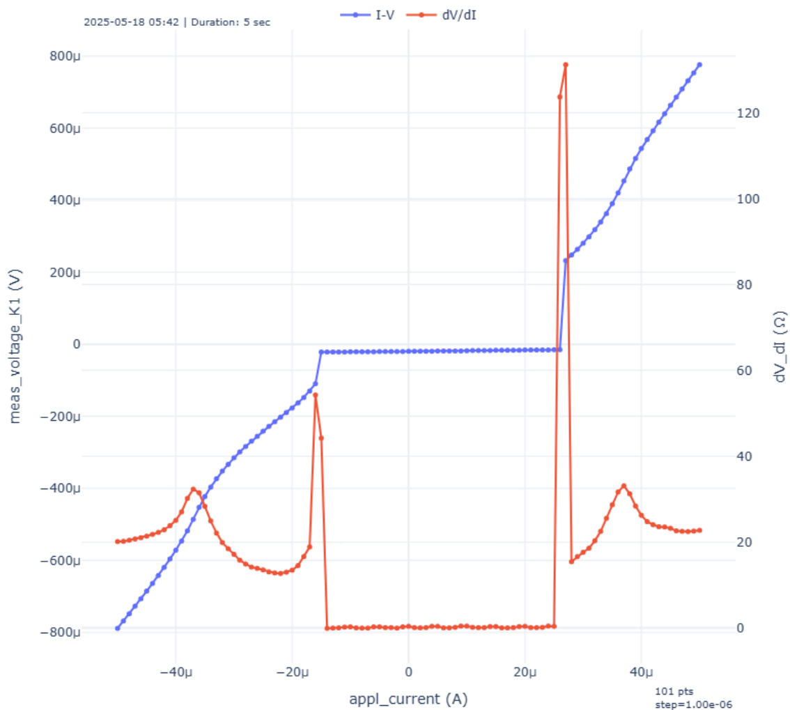
圖 7 PtTe 2 約瑟夫森接面的 MAR 特性
