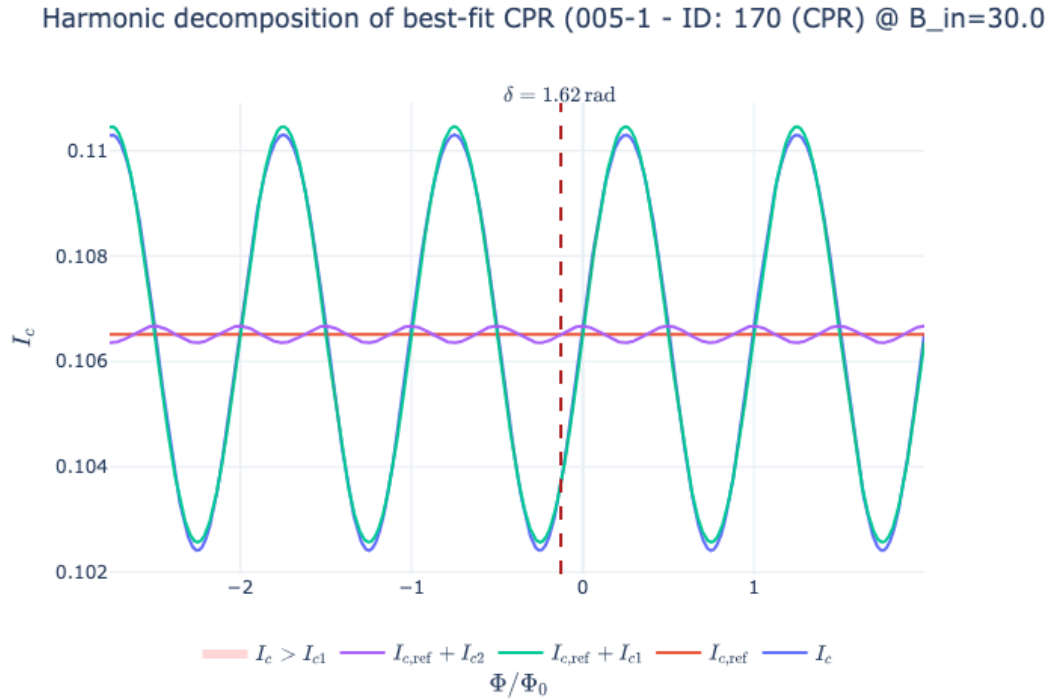
圖 18 重構的 PtTe 2 接面電流-相位關係 (Sample 005-1, Run 170)。實驗數據與擬合結果顯示了顯著的非正弦特徵。
