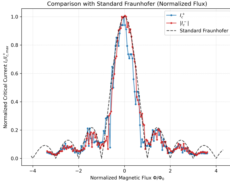
圖 12 標準夫朗和費干涉圖樣的正規化版本。左側圖顯示臨界電流隨正規化磁通量 ( \frac{\Phi}{\Phi_0} ) 的變化，其中 \frac{\Phi}{\Phi_0} = \frac{B_z' - B_{\text{offset}}}{B_{\text{period}}} 。 I_c 已除以 I_c^+ 的最大值進行正規化。正向臨界電流 I_c^+ 與負向臨界電流絕對值 |I_c^-| 在零場附近的行為顯示出高度的一致性。黑色虛線代
