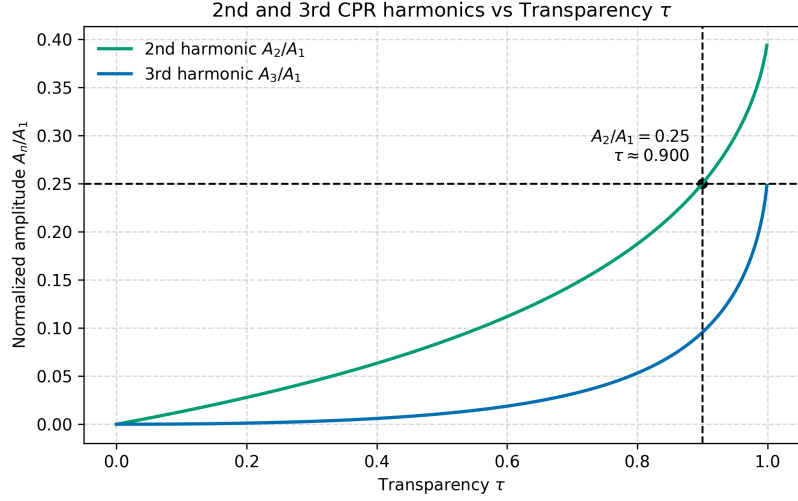
圖 16 二階與三階谐波分量隨透明度 \tau 的變化。為了產生 \frac{I_2}{I_1} = 0.25 的二階分量，透明度必須高達 \tau \approx 0.90 。
