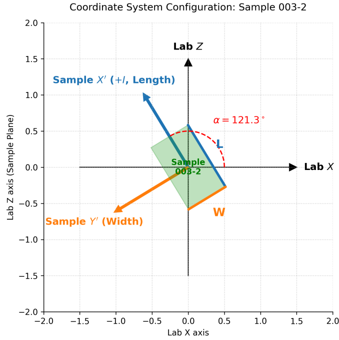
圖 9 Sample 003-2 的座標系配置示意圖。樣品位於實驗室 X-Z 平面，逆時針旋轉角度 \alpha = 121.3^\circ 。綠色矩形代表樣品，藍色箭頭指示沿長軸的電流方向（ x' axis）。
