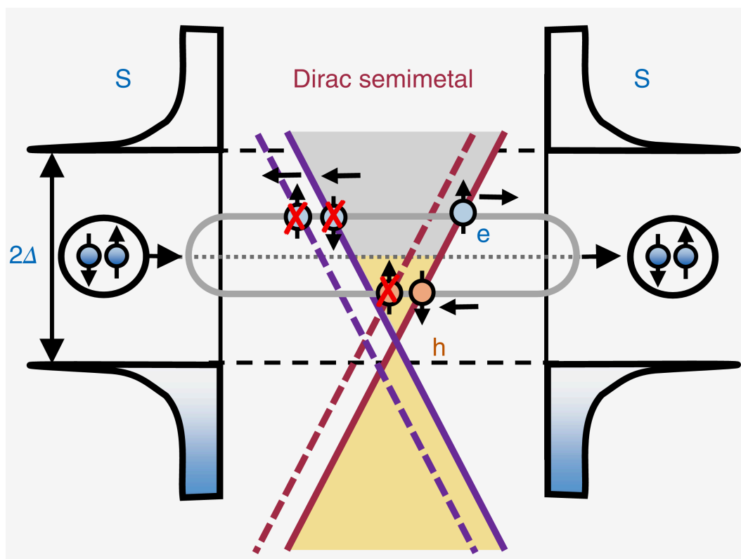
圖 3 S-DSM-S 約瑟夫森接面示意圖(Type-I)。Ref.[3]
