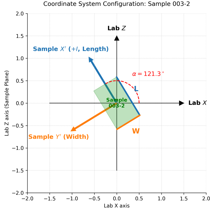
圖 8 Sample 003-2 的座標系配置示意圖。樣品位於實驗室 X-Z 平面，逆時針旋轉角度 \alpha = 121.3^\circ 。綠色矩形代表樣品，藍色箭頭指示沿長軸的電流方向 ( X' axis)。
