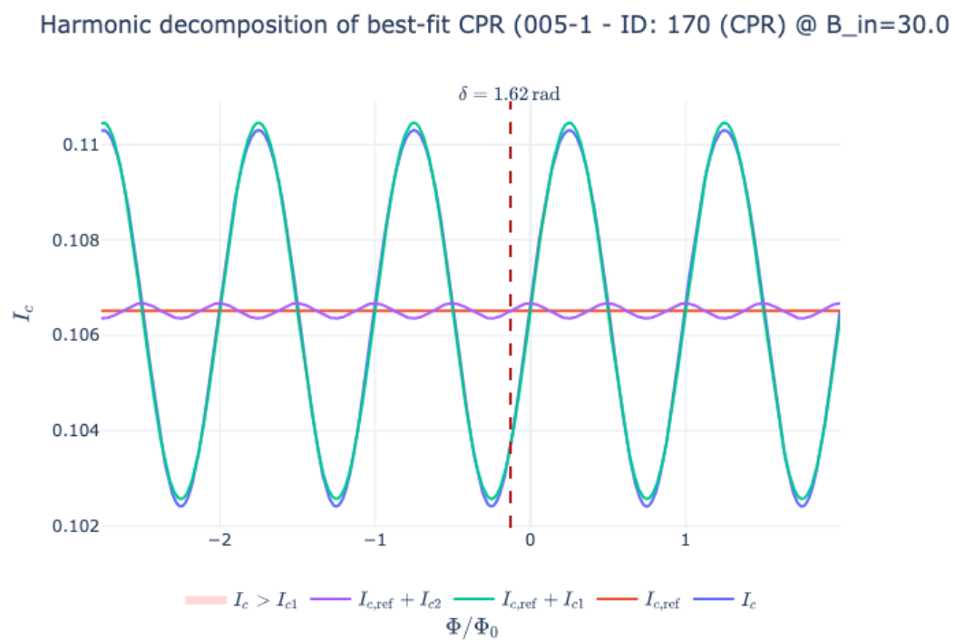
圖 15 重構的 \text{PtTe}_2 接面電流-相位關係 (Sample 005-1, Run 170)。實驗數據與擬合結果顯示了顯著的非正弦特徵。
