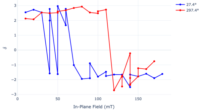
圖 19 Sample 003-2 在特定角度下的參數演化 (27.4° vs 297.4°)。(a) 臨界電流 I_c (b) 諧波比例 \frac{I_2}{I_1} (c) 一階諧波 I_1 (d) 二階諧波 I_2 (e) 相位偏移 \delta 藍色與紅色曲線分別代表
