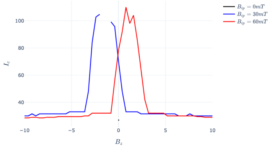
圖 12 面內磁場下夫朗和費圖樣的演化。隨著 B_{\text{in-plane}} 的增加，原本對稱的干涉圖樣逐漸變得不對稱，極小值位置發生偏移，包絡函數形狀也隨之改變。
