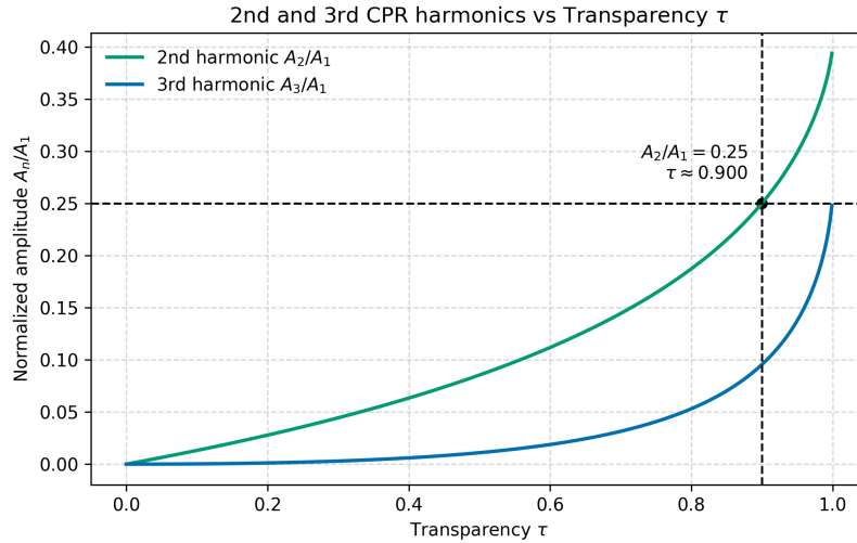
圖 13 二階與三階諧波分量隨透明度 \tau 的變化。為了產生 \frac{I_2}{I_1} = 0.25 的二階分量，透明度必須高達 \tau \approx 0.90 。
