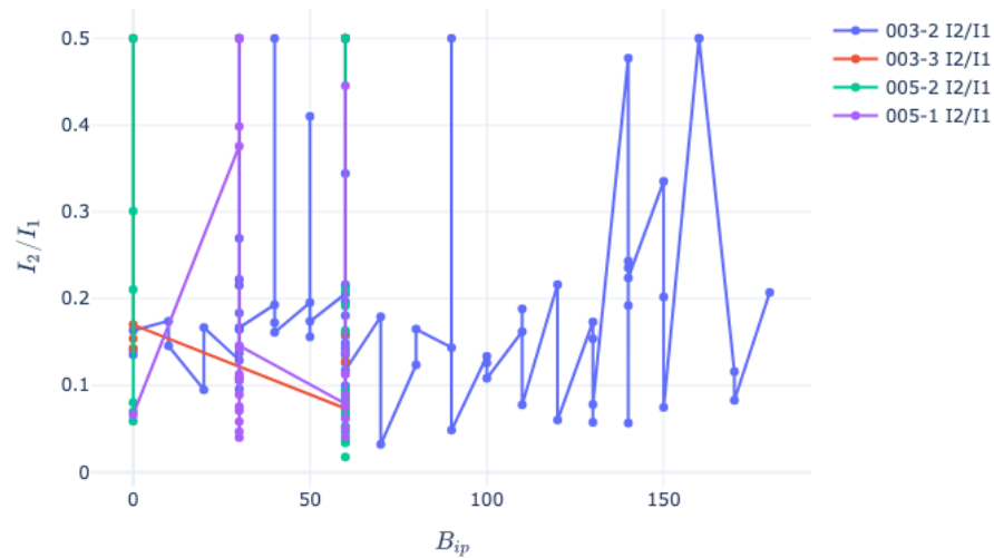
圖 17 二階諧波分量 ( \frac{I_2}{I_1} ) 隨面內磁場的演化。
