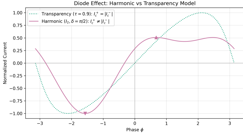
圖 14 透明度模型與諧波模型的比較。標準透明度模型 (綠線) 雖然能產生偏斜的波形，但仍保持 I_c^+ = |I_c^-| 的對稱性。含有相位偏移的諧波模型 (紫線) 則能自然描述
